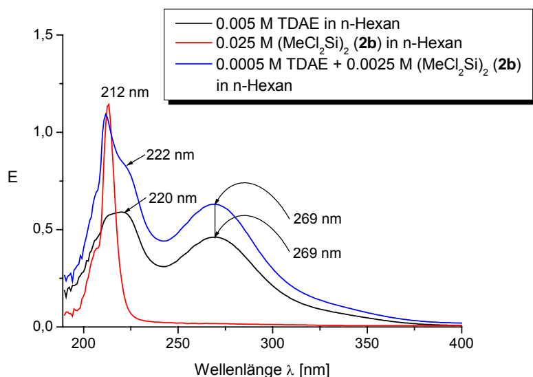
Abb. 13: UV/VIS-Spektren der Edukte TDAE und 1,1,2,2-Tetrachlorodimethyldisilan 2b und deren Mischung in n-Hexan (Meßbedingungen: 25 °C, 1 cm Suprasil-Quarzküvette)
