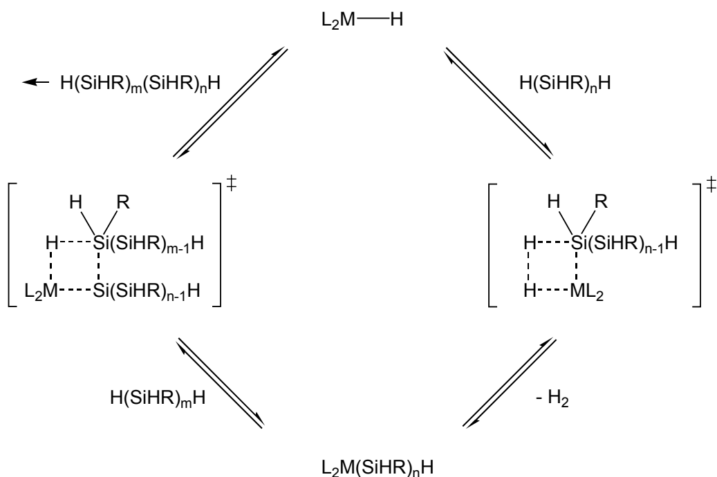
Schema 2: „ \sigma -bond metathesis mechanism“ nach T. D. Tilley [76,77]
