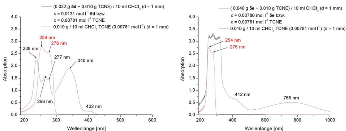
Abb. 42: UV/VIS-Spektren der Mischungen aus den fünfgliedrigen Heterocyclen 5d bzw. 5e und TCNE in CHCl 3 (Meßbedingungen: 1 mm Quarzküvette, Raumtemperatur)
