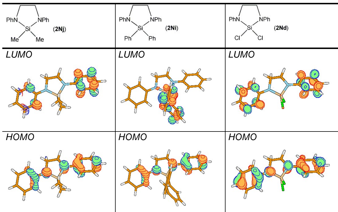
Abb. 28: Grenzorbitale der Diazasilimidazolidine 2Nj , 2Ni und 2Nd
