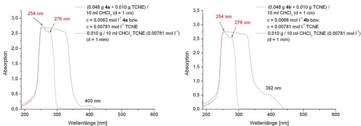
Abb. 47: UV/VIS-Spektren der Mischungen aus den Cyclotetrasilanen 4a bzw. 4b und TCNE in \text{CHCl}_3 (Meßbedingungen: 1 cm bzw. 1 mm Quarzküvette, Raumtemperatur)
