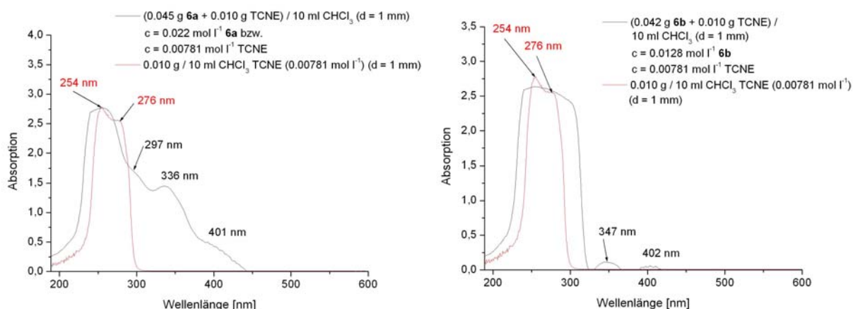
Abb. 43: UV/VIS-Spektren der Mischungen aus den sechsgliedrigen Heterocyclen 6a bzw. 6b und TCNE in CHCl 3 (Meßbedingungen: 1 mm Quarzküvette, Raumtemperatur)
