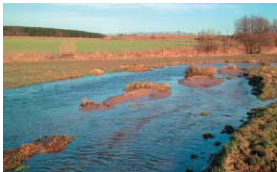
Abbildung B.24: Sandige Längsbänke und Tendenz zur Gerinneverzweigung (Hüseemann und Karthaus, 2004)
