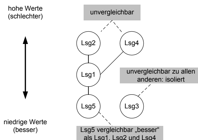
Abbildung 3.10: Hassediagramm (Heinrich, 2001)
