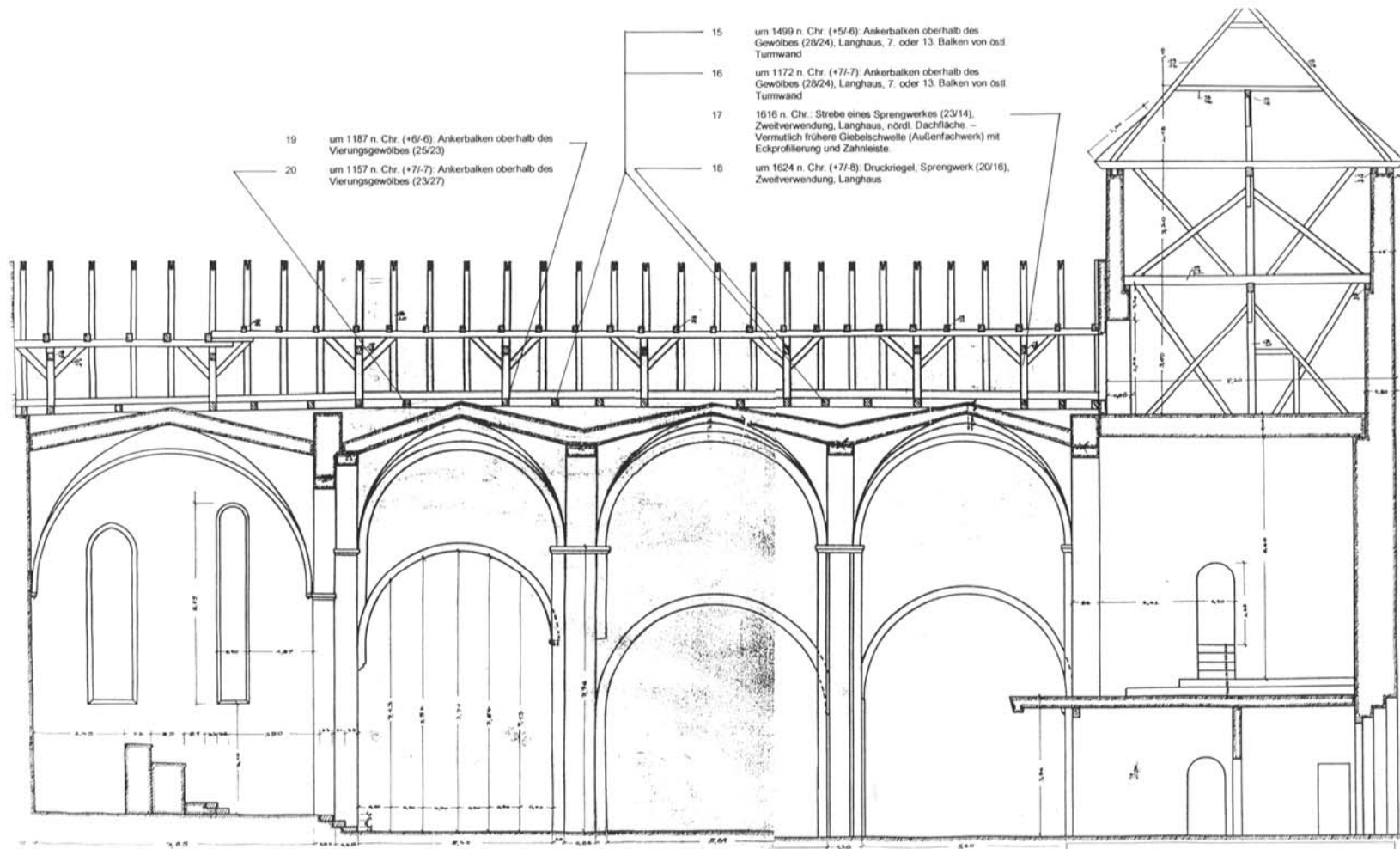
ST. KILIAN - HÖXTER Längsschnitt, Blickrichtung nach Süden Bauaufnahme durch Studenten der Baugewerkschule Höxter 15.02.1951, NW Staatsarchiv Detmold D73Tit.4Nr.3200 mit Eintragungen zu Baubefunden M+100 o. M. Bearbeitung: Heiko Seidel 09/2001
