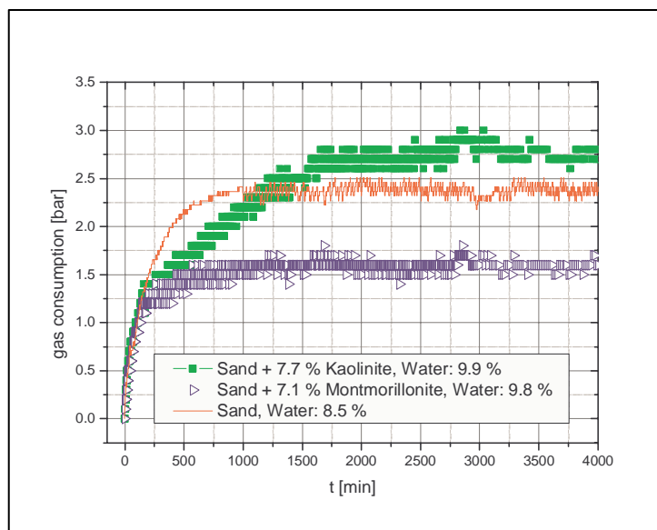
Abbildung 1. Zeitlicher Verlauf der Methan-Aufnahme in synthetischen Sedimenten verschiedener Zusammensetzung; die geringere Gasaufnahme in Montmorillonit-haltigen Sedimenten ist durch die Wasseraufnahme des zuvor getrockneten Montmorillonits verursacht.
