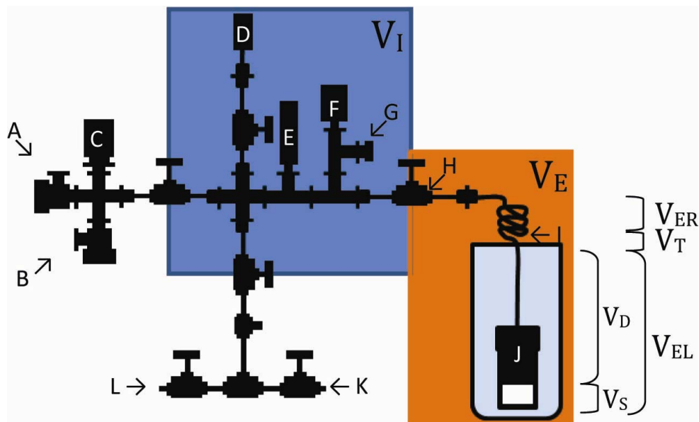
Abbildung 2. BET-Apparatur mit initialem Gasvolumen V_I und dem expandierten zusätzlichen Volumen V_E . Aus dem Druckabfall bei Öffnen des Ventils H lässt sich unter Kenntnis der übrigen Volumina ( V_{ER} , V_T , V_D und V_S ) und der Probenmasse die spezifische Oberfläche und die Adsorptionsenergie berechnen. Mehrfache Modifikationen des Probenbehälters J und der relativen Volumina waren notwendig bis zur Durchführung von routinemäßige Messungen.
