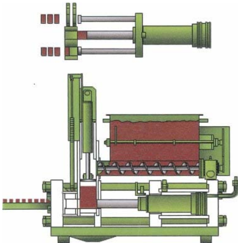
Bild 10: Spänepresse Fabrikat RUF
