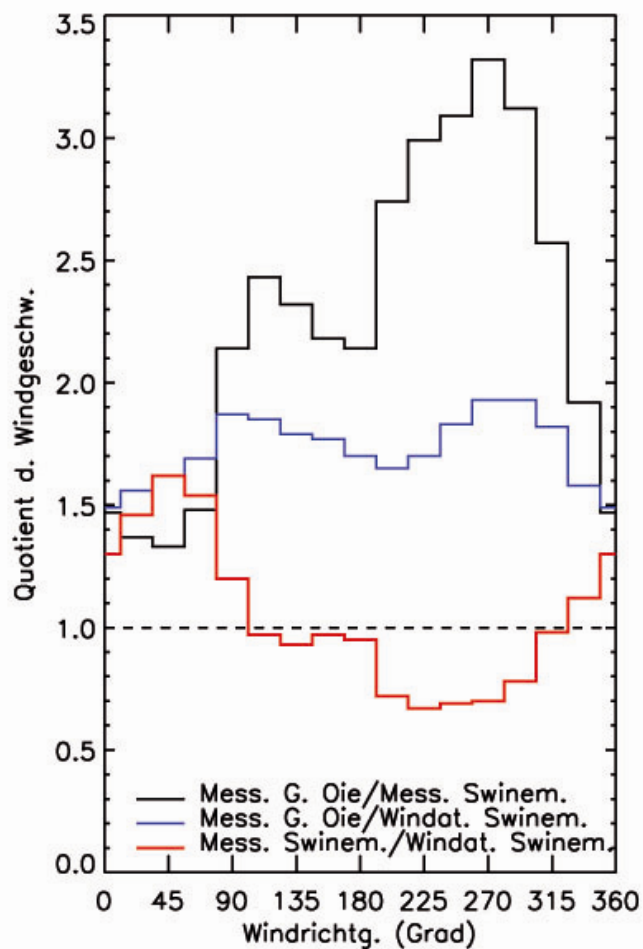
Abb. 3.8.b: Quotienten der Mittelwerte der Windgeschwindigkeiten für die 16 Windrichtungsklassen für gemessene und mit dem Windatlas berechnete Zeitreihen. Eingangspunkt für Windatlasrechnungen: Darßer Schwelle. Bezugszeitraum: 1.1.2002 bis 31.12.2005
