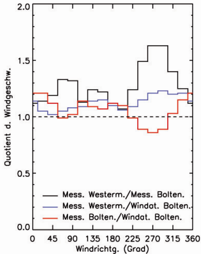
Abb. 3.5.b: Quotienten der Mittelwerte der Windgeschwindigkeiten für die 16 Windrichtungsklassen für gemessene und mit dem Windatlas berechnete Zeitreihen. Eingangspunkt für Windatlasrechnungen: Westermarkelsdorf. Bezugszeitraum: 1.11.1996 bis 31.10.2005.
