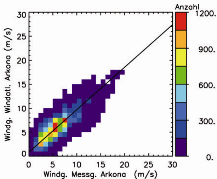
Abb. 3.7.a: Korrelation zwischen den Windgeschwindigkeiten, die in Arkona gemessen (Abszisse) und mit dem Windatlas für Arkona berechnet wurden (Ordinate). Eingabewerte für die Windatlas-Rechnungen: an der Darßer Schwelle gemessene Windgeschwindigkeiten. Durchgezogene Linie: Ausgleichsgerade. Bezugszeitraum: 1.9.2001 bis 31.8.2005.
