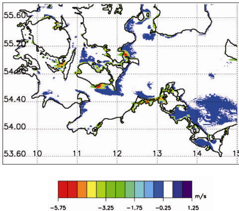
Abb. 3.2: Differenz der Windgeschwindigkeit in 10 m Höhe, berechnet bei Wasserständen von 2 m unter NN und 0 m NN. (Windgeschwindigkeiten bei 0 m NN - Windgeschwindigkeiten bei 2 m unter NN). Windfelder berechnet mit einer Windrichtung von 90 Grad und einer Windgeschwindigkeit von 35 m/s in der Nähe der Darßer Schwelle.
