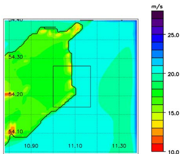
Abb. 4.4: Mit dem MKW und den Randwerten aus den interpolierten COSMO-EU-Windfeldern berechnete Windgeschwindigkeiten im Gebiet um Dahme. In 300 m Höhe wurden eine feste Windgeschwindigkeit von 29.6 m/s und eine Windrichtung von 56.7 Grad vorgegeben.
