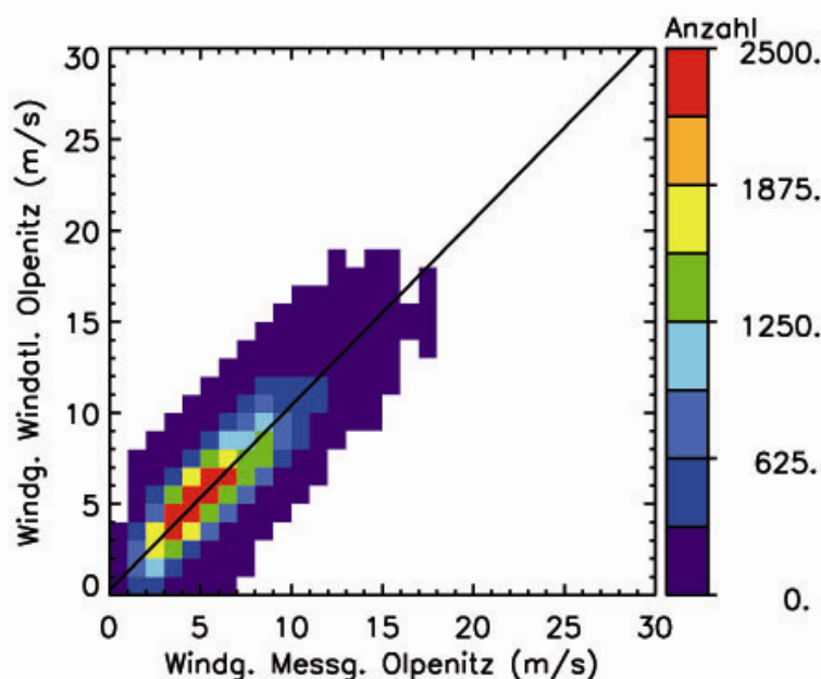
Abb. 3.4.a: Korrelation zwischen den Windgeschwindigkeiten, die in Olpenitz gemessen (Abszisse) und mit dem Windatlas für Olpenitz berechnet wurden (Ordinate). Eingabewerte für die Windatlas-Rechnungen: am Leuchtturm Kiel gemessene Windgeschwindigkeiten. Durchgezogene Linie: Ausgleichsgerade. Bezugszeitraum: 1.11.1996 bis 31.10.2005
