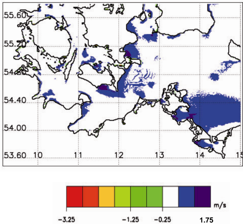
Abb. 3.1: Differenz der Windgeschwindigkeit in 10 m Höhe, berechnet bei Wasserständen von 3 m über NN und 0 m NN (Windgeschwindigkeiten bei 3 m über NN - Windgeschwindigkeiten bei 0 m NN). Windfelder berechnet mit einer Windrichtung von 90 Grad und einer Windgeschwindigkeit von 35 m/s in der Nähe der Darßer Schwelle.
