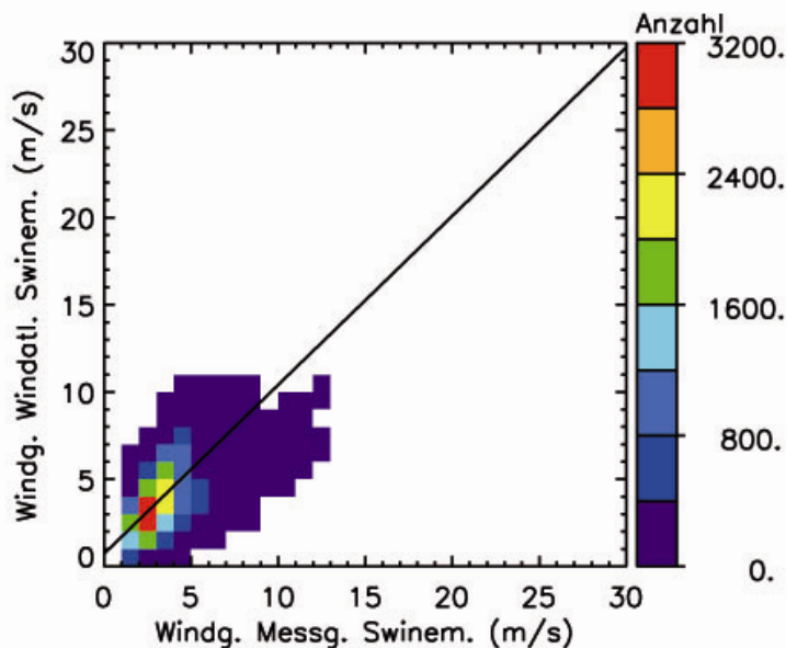
Abb. 3.8.a: Korrelation zwischen den Windgeschwindigkeiten, die in Swinemünde gemessen (Abszisse) und mit dem Windatlas für Swinemünde berechnet wurden (Ordinate). Eingabewerte für die Windatlas-Rechnungen: an der Darßer Schwelle gemessene Windgeschwindigkeiten. Durchgezogene Linie: Ausgleichsgerade. Bezugszeitraum: 1.1.2002 bis 31.12.2005
