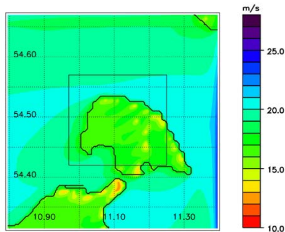
Abb. 4.2: Mit dem MKW und den Randwerten aus den interpolierten COSMO-EU-Windfeldern berechnete Windgeschwindigkeiten im Gebiet um Fehmarn. In 300 m Höhe wurden eine feste Windgeschwindigkeit von 29.6 m/s und eine Windrichtung von 57 Grad vorgegeben.
