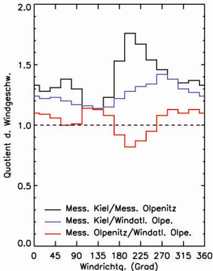
Abb. 3.4.b: Quotienten der Mittelwerte der Windgeschwindigkeiten für die 16 Windrichtungsklassen für gemessene und mit dem Windatlas berechnete Zeitreihen. Eingangspunkt für Windatlasrechnungen: Kiel. Bezugszeitraum: 1.11.1996 bis 31.10.2005
