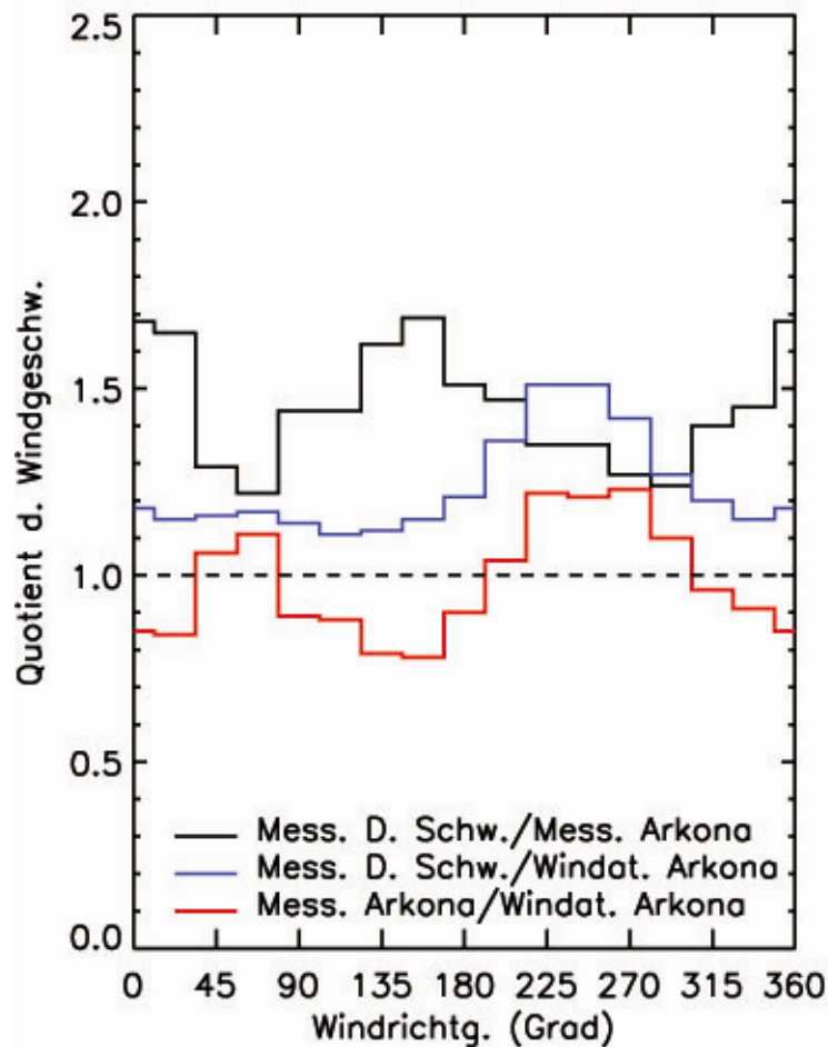
Abb. 3.7.b: Quotienten der Mittelwerte der Windgeschwindigkeiten für die 16 Windrichtungsklassen für gemessene und mit dem Windatlas berechnete Zeitreihen. Eingangspunkt für Windatlasrechnungen: Darßer Schwelle. Bezugszeitraum: 1.9.2001 bis 31.8.2005
