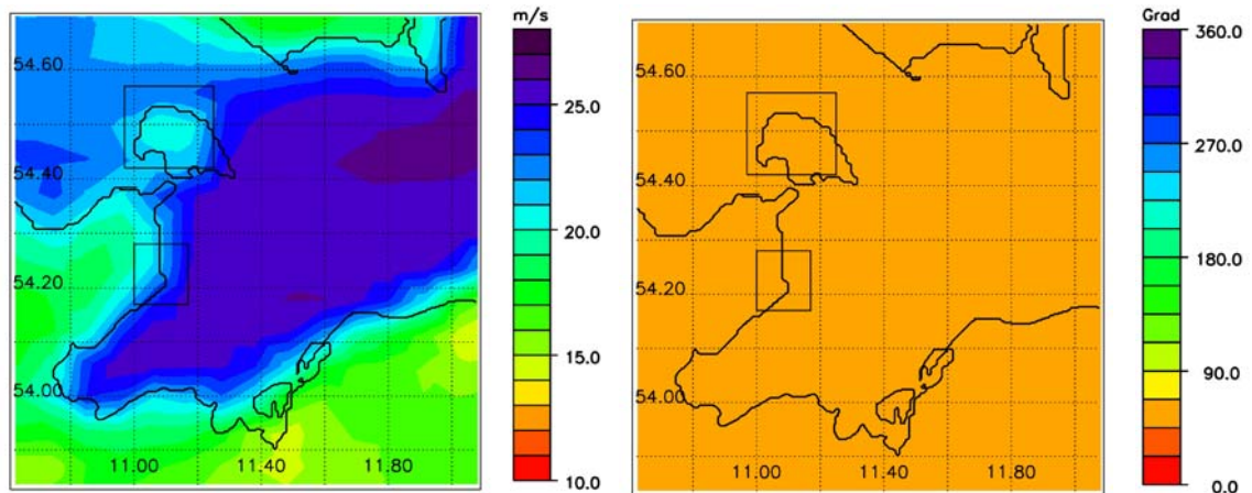
Abb. 4.1: Von der COSMO-EU-Vorhersage auf das MKW-Gitter interpolierte Windgeschwindigkeitsfeld (linke Abb.) und Windrichtungen (rechte Abb.) am 17.10.2003, 12 UTC + 178 Stunden Vorhersage in 10 m Höhe über NN bzw. über Grund im Windatlas-Gebiet Mecklenburger Bucht. Die markierten Rechtecke beschreiben die Untersuchungsgebiete Fehmarn und Dahme.
