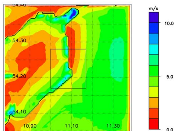
Abb. 4.5: Mit dem COSMO-EU bestimmte Windgeschwindigkeiten in 10 m Höhe (Abb. 4.1) minus der mit dem MKW berechneten Geschwindigkeiten (Abb. 4.4).
