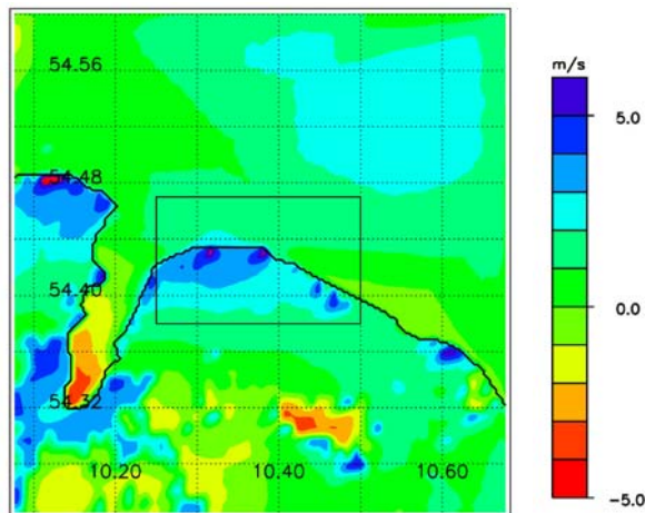
Abb. 4.8: Mit dem COSMO-EU berechnete Windgeschwindigkeiten in 10 m Höhe (Abb. 4.6) minus mit dem MKW berechnete Geschwindigkeiten (Abb. 4.7).
