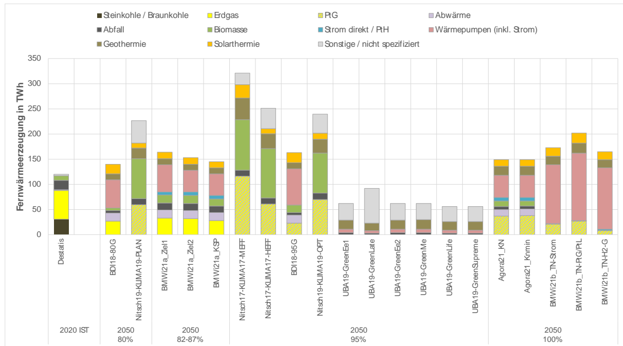
Abbildung 11: Fernwärmeerzeugung nach Energieträgern im Szenarienvergleich. Quelle für IST-Daten von 2020: (Statistisches Bundesamt, 2021a, 2021b).
