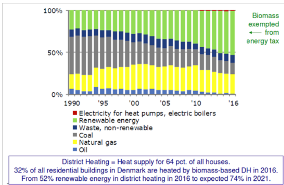
Abbildung 5: Entwicklung des Brennstoff- bzw. Energiemixes in der Fernwärmeversorgung Dänemarks im Zeitraum von 1990 bis heute. Quelle: Ole Odgaard, Danish Energy Agency.
