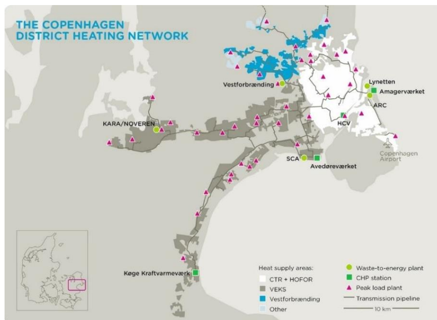
Abbildung 4: Übersicht über den Fernwärmeverbund im Großraum Kopenhagen. Quelle: Morten Duedahl, DBDH.
