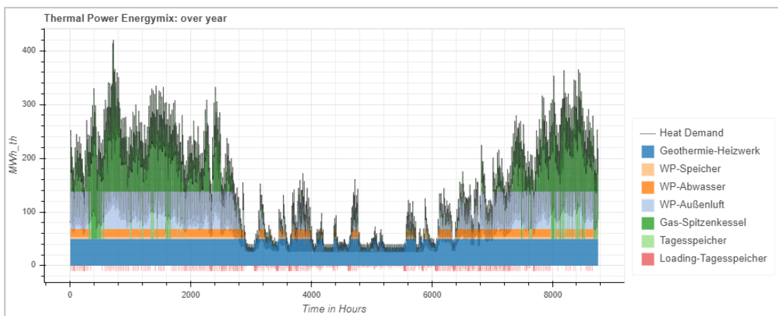
Abbildung 145: Jahresganglinie für das System der Wärmebedarfsstufe 900 GWh.
