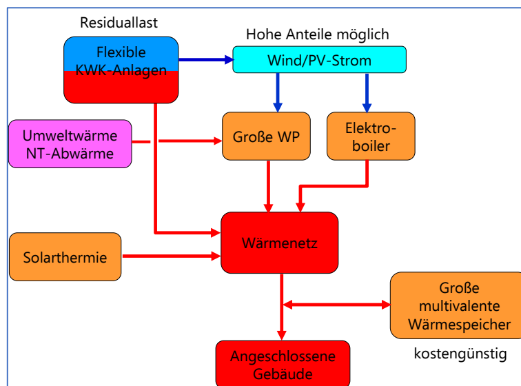
Abbildung 212: Flexibilitätsoptionen für die Stromerzeugung durch Wärmenetze und große thermische Speicher.
