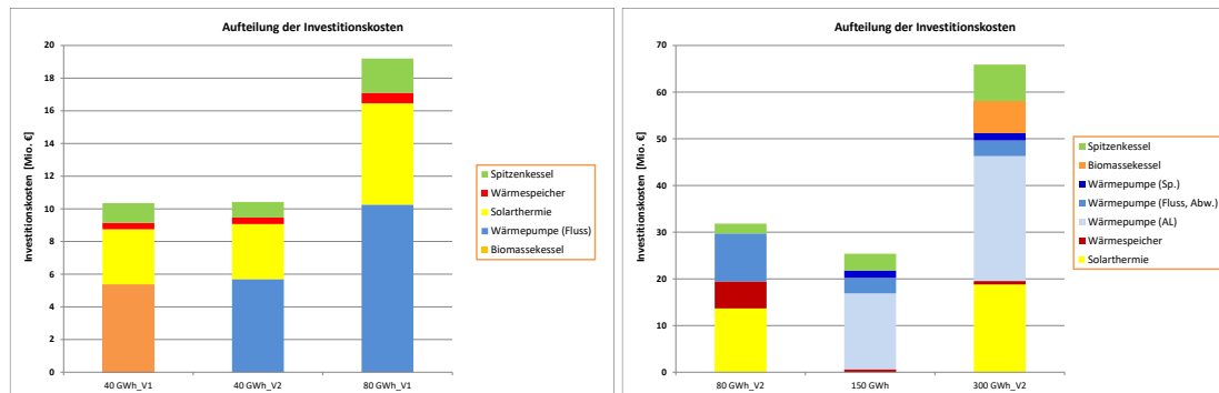
Abbildung 148: Verteilung der Investitionskosten auf die verschiedenen Komponenten.
