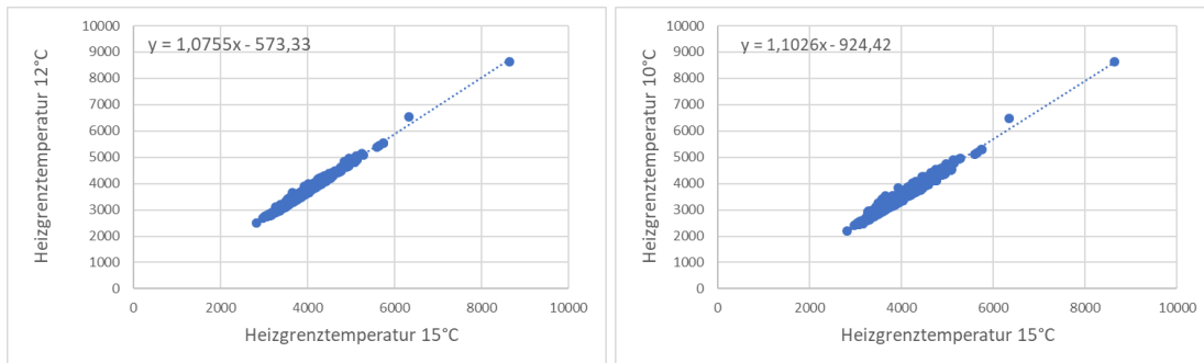
Abbildung 27: Umwandlungsfunktionen zwischen den verschiedenen Heizgrenztemperaturen der Gradtagszahlen.
