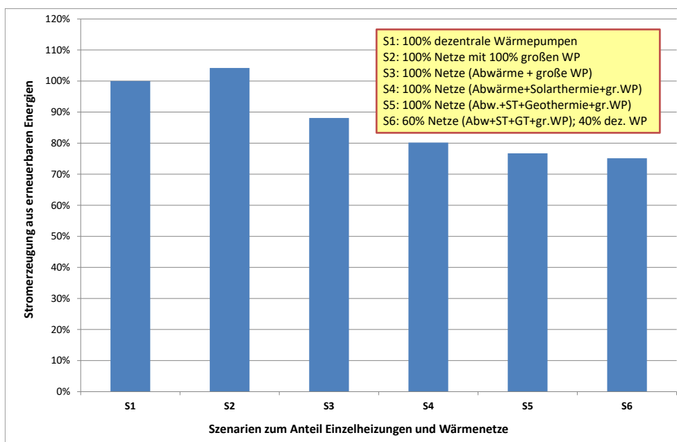
Abbildung 214: Strombedarf aus erneuerbaren Energien in Abhängigkeit des Anteils dezentraler Wärmepumpen und Wärmenetze.
