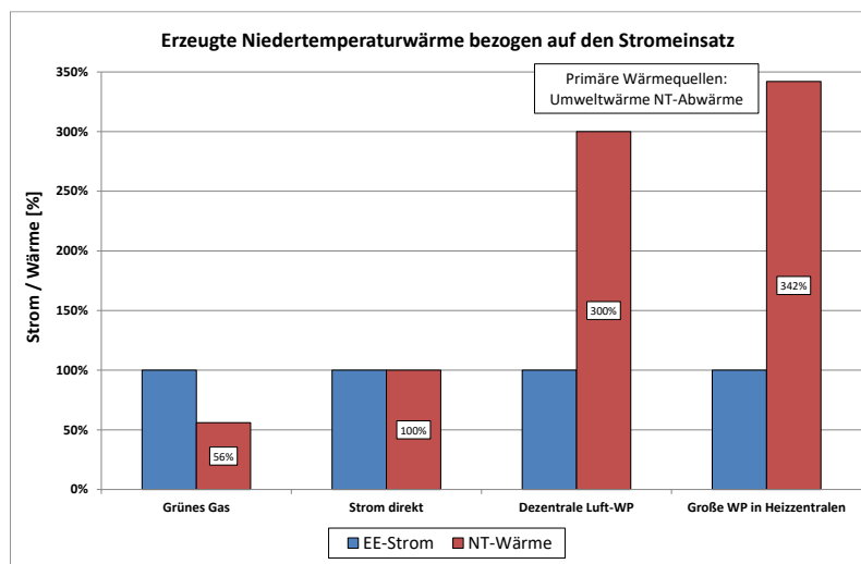
Abbildung 211: Erzeuge Niedertemperaturwärme bezogen auf den Einsatz von regenerativem Strom im Vergleich der drei Umwandlungsketten.
