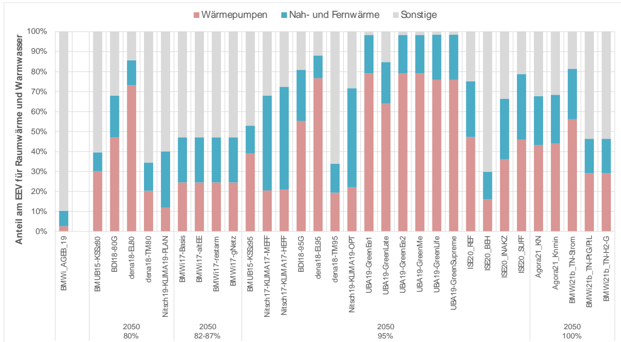
Abbildung 10: Anteile der Schlüsseltechnologien Wärmepumpen und Nah-/Fernwärme am EEV für Raumwärme und Warmwasser 5 .
