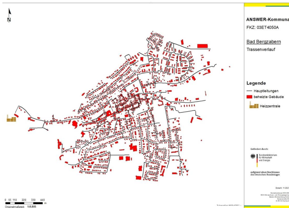
Abbildung 190: Mit GIS-Methoden berechnete Netztrassen und beheizte Gebäude in der Stadt Bad Bergzabern.
