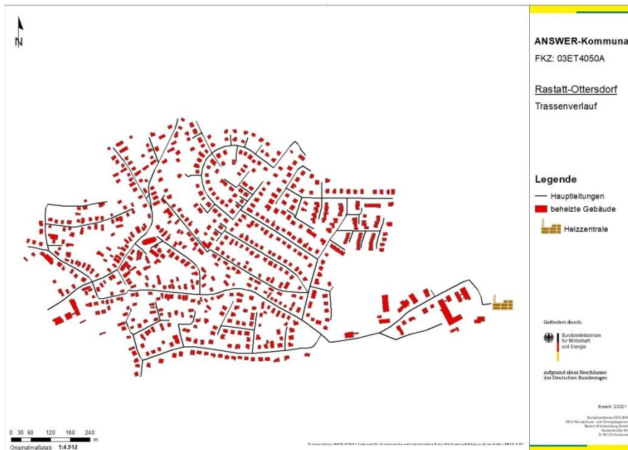
Abbildung 95: Beheizte Gebäude und Trassenverlauf der Hauptleitungen in Rastatt-Ottersdorf.
