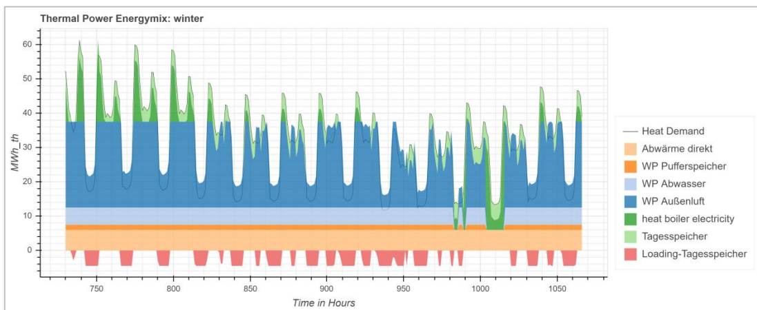
Abbildung 143: 150 GWh: Ganglinie für einen Zeitraum von zwei Wochen im Winter.
