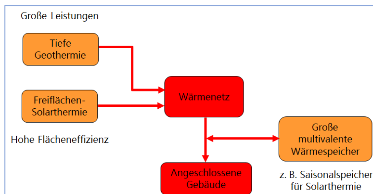
Abbildung 213: Einbindung von großer Solarthermie und tiefer Geothermie in Wärmenetze.
