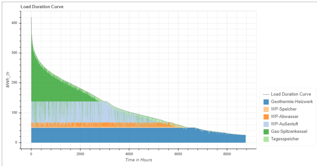
Abbildung 146: Jahresdauerlinie für das System der Wärmebedarfsstufe 900 GWh.
