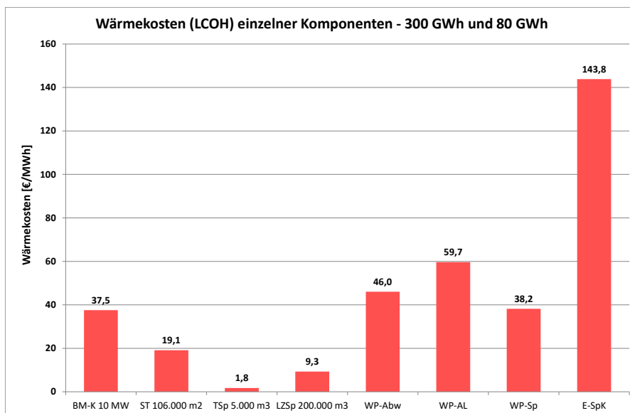
Abbildung 150: Wärmekosten (Levelized cost of heat) einzelner Komponenten.
