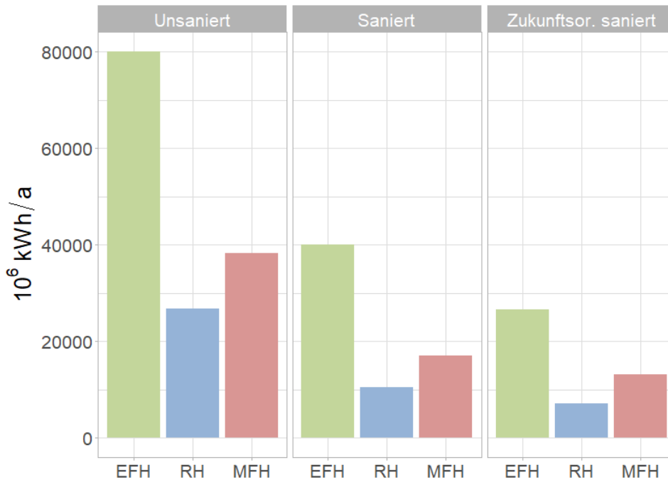
Abbildung 32: Wärmebedarf für Baden-Württemberg je nach Gebäudetyp und Sanierungsszenario für das Bauteilverfahren.
