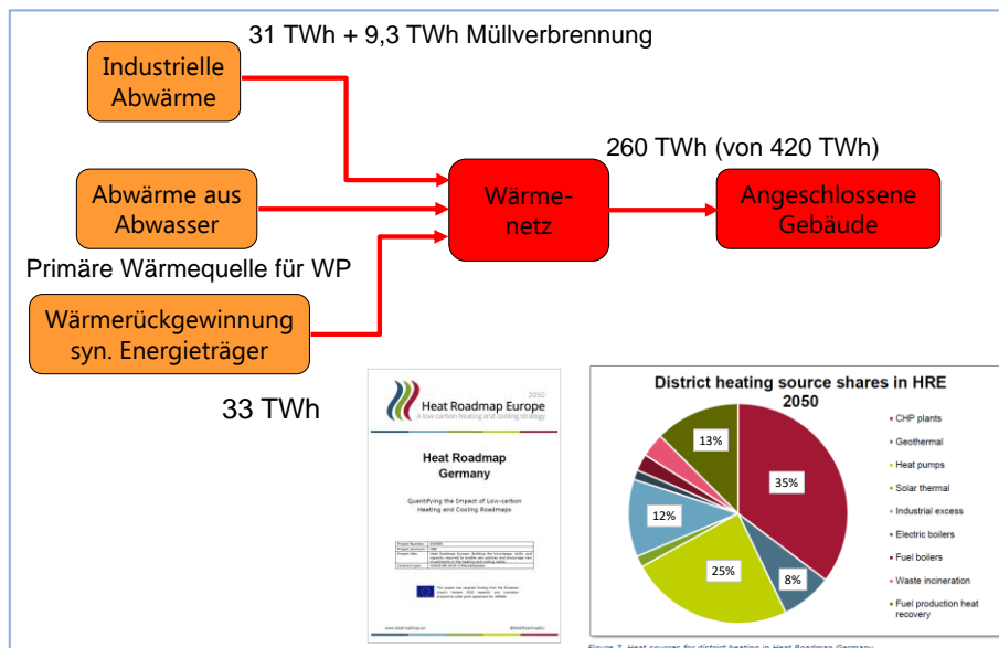
Abbildung 209: Steigerung der strukturellen Effizienz über Abwärmenutzung mit Hilfe von Wärmenetzen. Zahlbeispiel: Heat Roadmap Germany (Paardekooper, 2018)-
