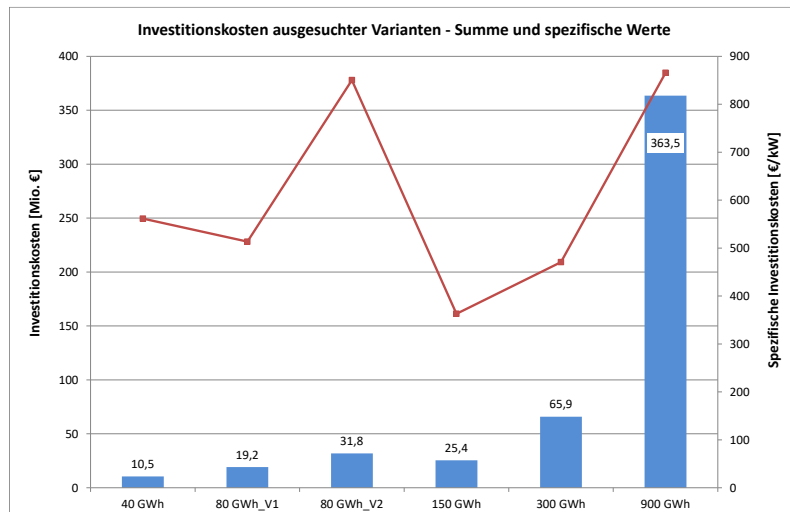
Abbildung 147: Überblick über die aufsummierten und spezifischen Investitionskosten der verschiedenen Systeme.
