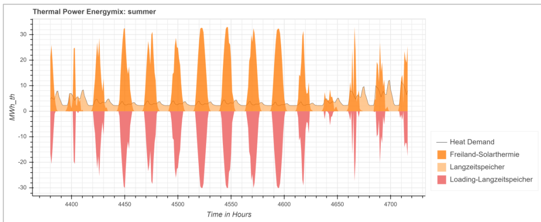
Abbildung 141: 80 GWh_V2: Ganglinie für einen Zeitraum von zwei Wochen im Sommer.
