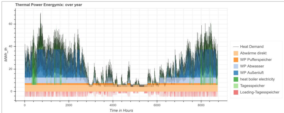
Abbildung 142: Jahresganglinie für das System der Wärmebedarfsstufe 150 GWh.
