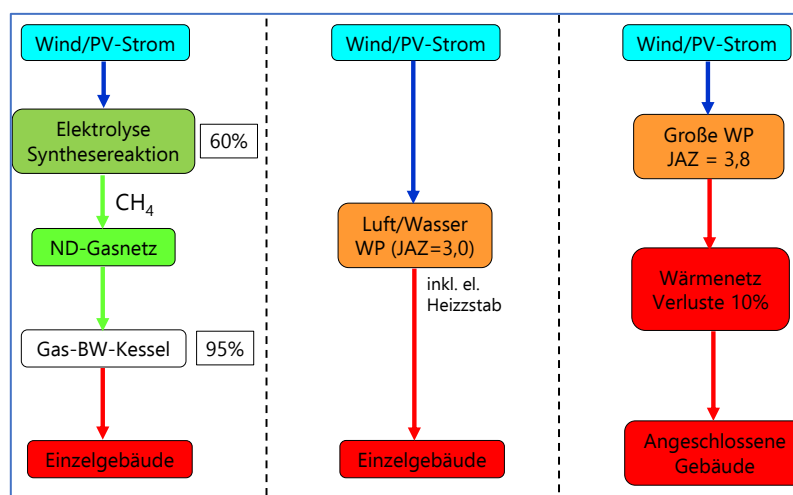
Abbildung 210: Aufbau und Vergleich verschiedener Umwandlungsketten zur Nutzung von erneuerbarem Strom in der Wärmeversorgung.
