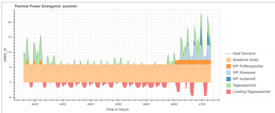
Abbildung 144: 150 GWh: Ganglinie für einen Zeitraum von zwei Wochen im Sommer.
