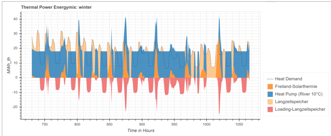
Abbildung 140: 80 GWh_V2: Ganglinie für einen Zeitraum von zwei Wochen im Winter.
