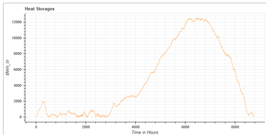
Abbildung 139: 80 GWh_V2: Jahresganglinie zur Beladung des Langzeitwärmespeichers.
