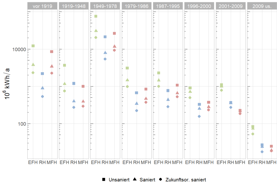
Abbildung 33: Wärmebedarf je nach Bauperiode unterschieden in Gebäudetyp und Sanierungsszenario.
