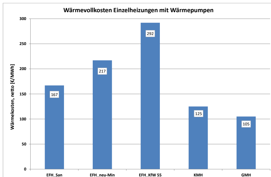
Abbildung 151: Wärmevollkosten für Einzelheizungen mit Wärmepumpen.
