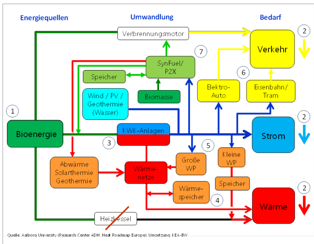
Abbildung 208: Struktur des Energiesystems mit 100 % erneuerbaren Energien und einer starken Kopplung zwischen den Sektoren (Smart Energy System).
