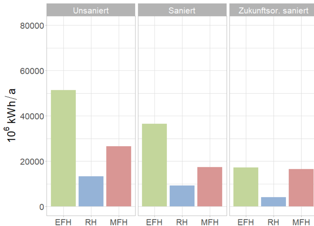
Abbildung 29: Wärmebedarf für Baden-Württemberg je nach Gebäudetyp und Sanierungsszenario für das Kennwertverfahren.
