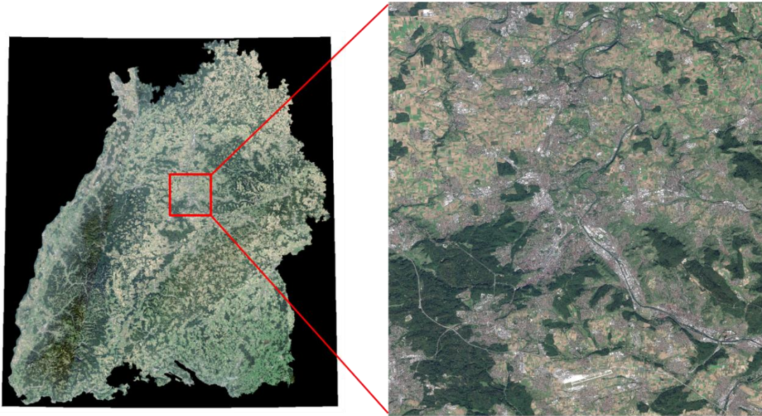
Abbildung 16: Sentinel-2 Mosaik von Baden-Württemberg (links) mit einem Ausschnitt von Stuttgart (rechts).
