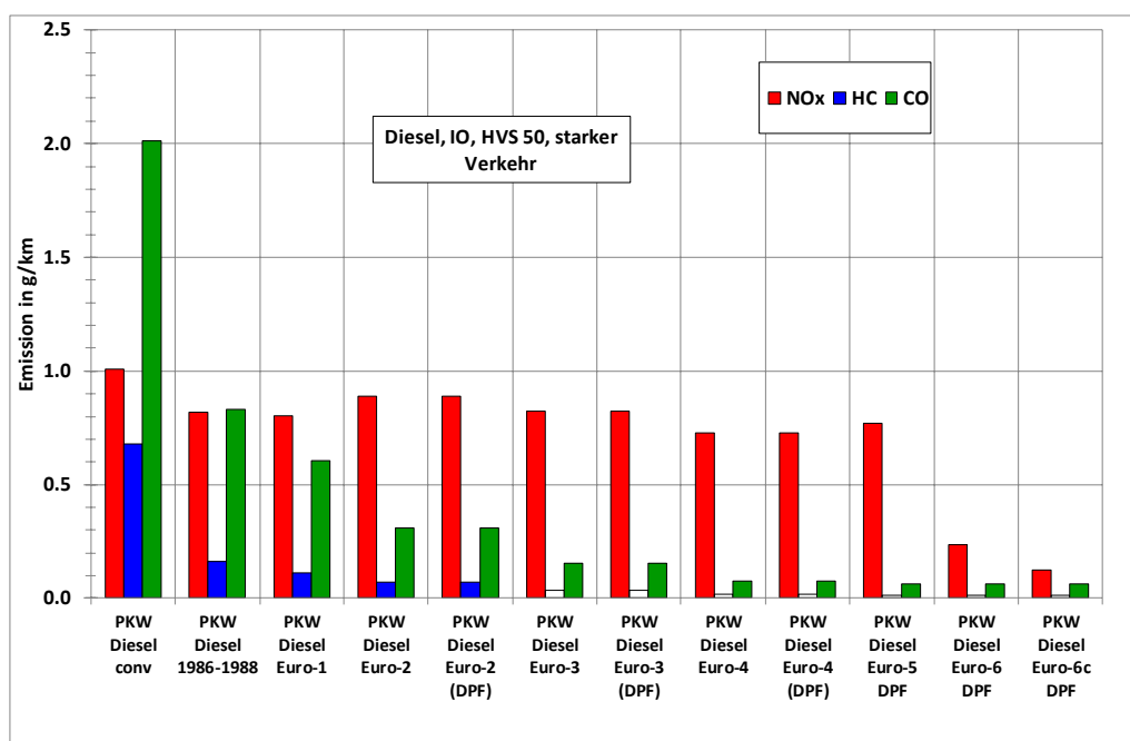
Abb. 6-5: Emissionsfaktoren der Handbuch-Fahrzeugschichten mit Dieselmotor für NO x , HC und CO /13/
