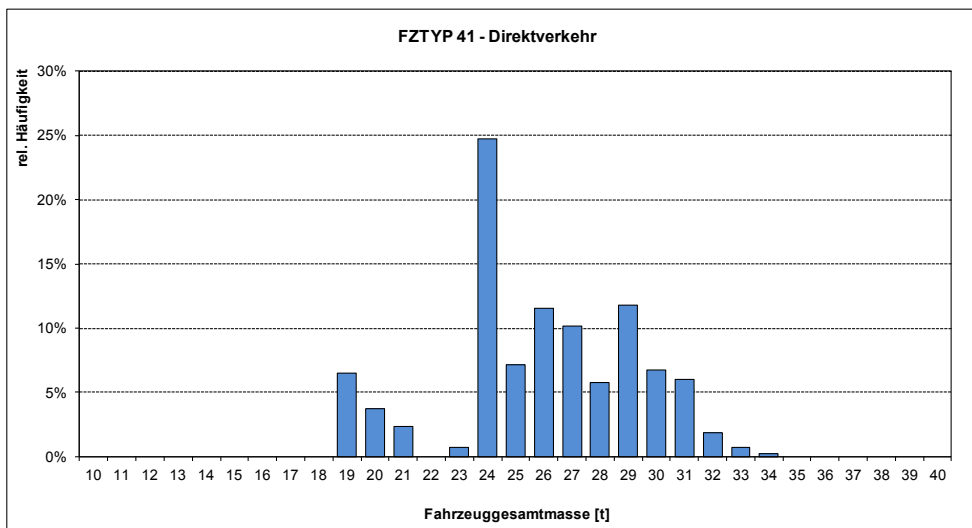
Abb. 75: Verteilung der Fahrzeugesamtmassen äquivalenter Lkw zu Lang-Lkw Typ 1, Fahrzeugtyp 41
