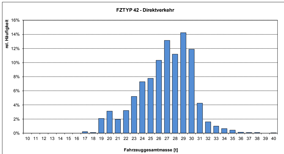
Abb. 10: Verteilung der Fahrzeugesamtmassen äquivalenter Lkw, Fahrzeugtyp 42 im Direktverkehr
