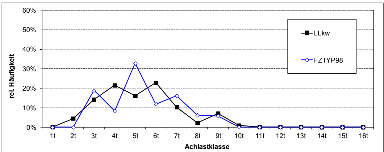
Abb. 50: Verteilungsfunktionen der Lang-Lkw und äquivalenten konventionellen Lkw des Unternehmens U34 (Direktverkehr)
