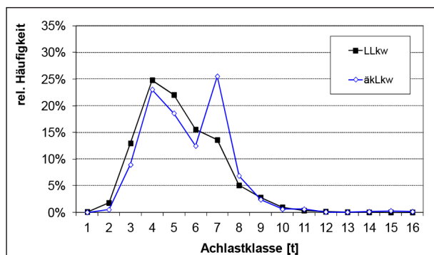
Bild 14: Achslastverteilung von Lang-Lkw und äquivalenten konventionellen Lkw im Direktverkehr
