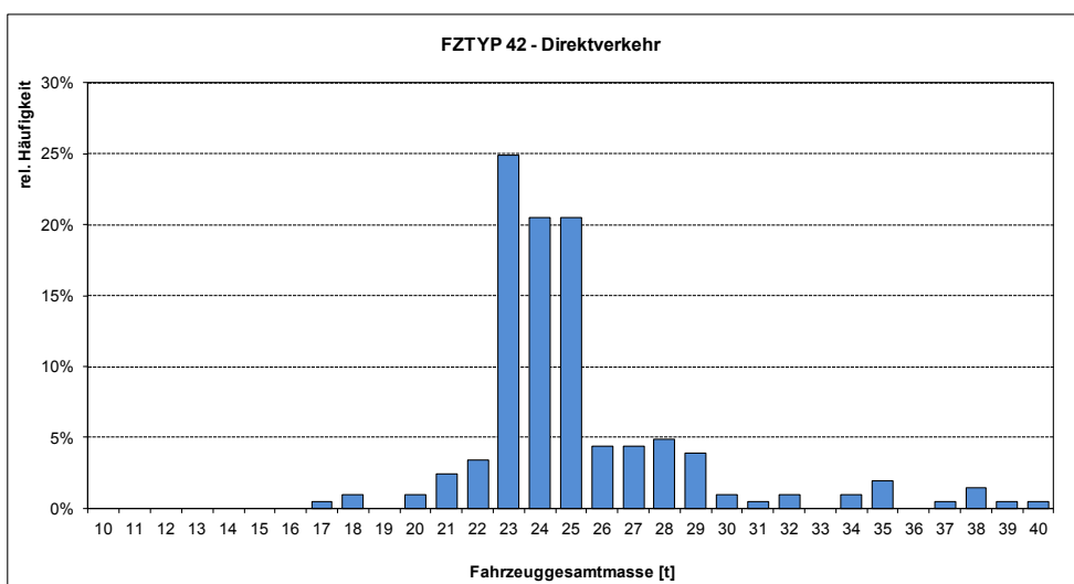
Abb. 76: Verteilung der Fahrzeugesamtmassen äquivalenter Lkw zu Lang-Lkw Typ 1, Fahrzeugtyp 42
