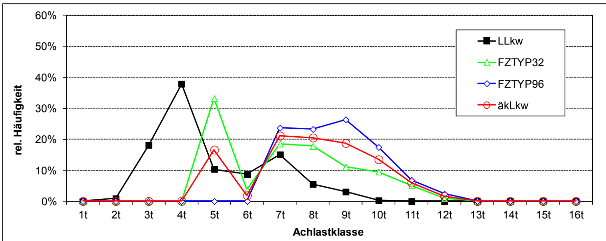
Abb. 46: Verteilungsfunktionen der Lang-Lkw und äquivalenten konventionellen Lkw des Unternehmens U31 (Direktverkehr)
