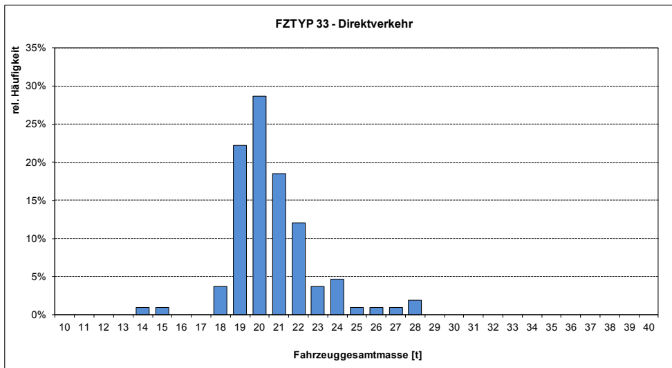
Abb. 74: Verteilung der Fahrzeugesamtmassen äquivalenter Lkw zu Lang-Lkw Typ 1, Fahrzeugtyp 33
