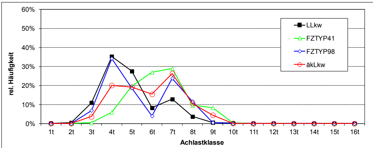
Abb. 40: Verteilungsfunktionen der Lang-Lkw und äquivalenten konventionellen Lkw des Unternehmens U24 (Direktverkehr)
