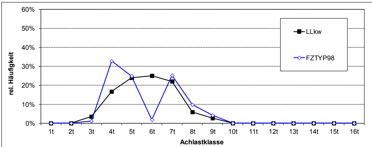
Abb. 34: Verteilungsfunktionen der Lang-Lkw und äquivalenten konventionellen Lkw des Unternehmens U17 (Direktverkehr)
