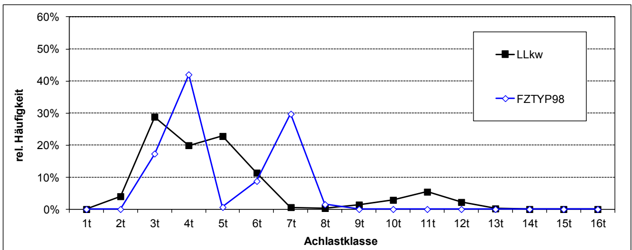
Abb. 21: Verteilungsfunktionen der Lang-Lkw und äquivalenten konventionellen Lkw des Unternehmens U6 (Direktverkehr)
