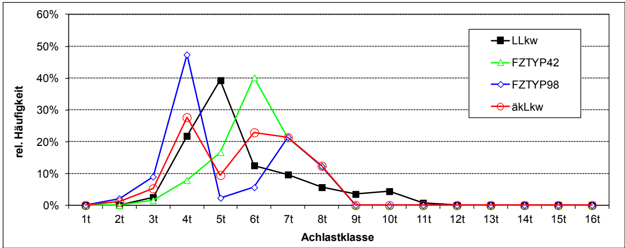
Abb. 42: Verteilungsfunktionen der Lang-Lkw und äquivalenten konventionellen Lkw des Unternehmens U26 (Direktverkehr)
