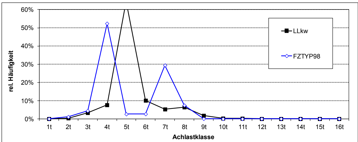
Abb. 44: Verteilungsfunktionen der Lang-Lkw und äquivalenten konventionellen Lkw des Unternehmens U29 (Direktverkehr)
