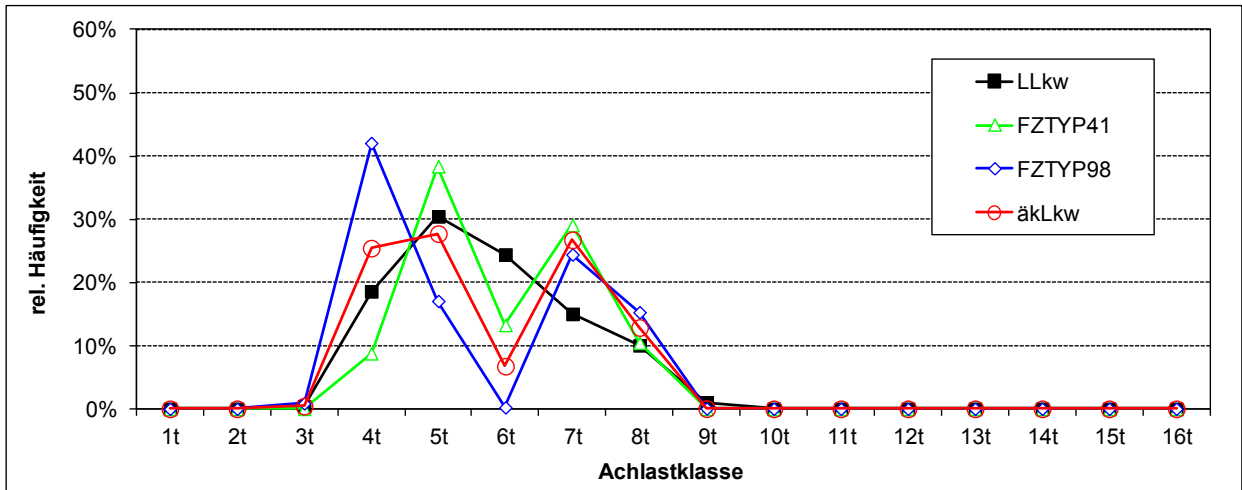
Abb. 61: Verteilungsfunktionen der Lang-Lkw und äquivalenten konventionellen Lkw des Unternehmens U45 (Direktverkehr)
