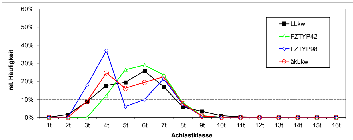
Abb. 23: Verteilungsfunktionen der Lang-Lkw und äquivalenten konventionellen Lkw des Unternehmens U8 (Direktverkehr)
