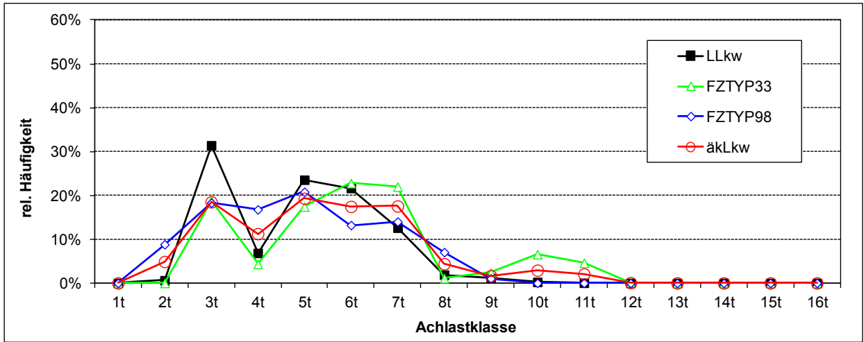
Abb. 19: Verteilungsfunktionen der Lang-Lkw und äquivalenten konventionellen Lkw des Unternehmens U4 (Direktverkehr)
