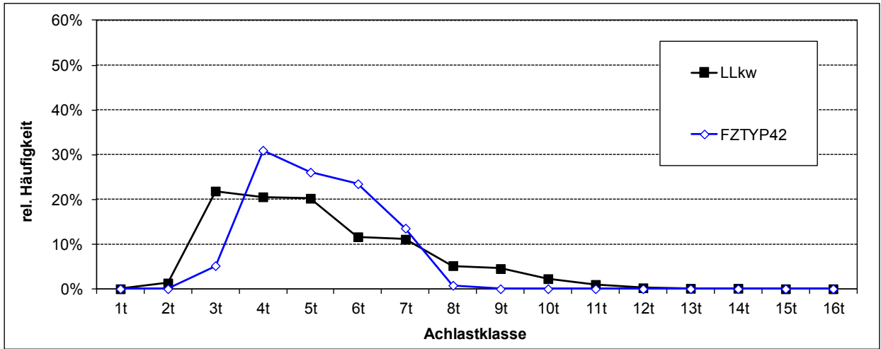
Abb. 48: Verteilungsfunktionen der Lang-Lkw und äquivalenten konventionellen Lkw des Unternehmens U32, Typ 5 mit 6 Achsen (Direktverkehr)
