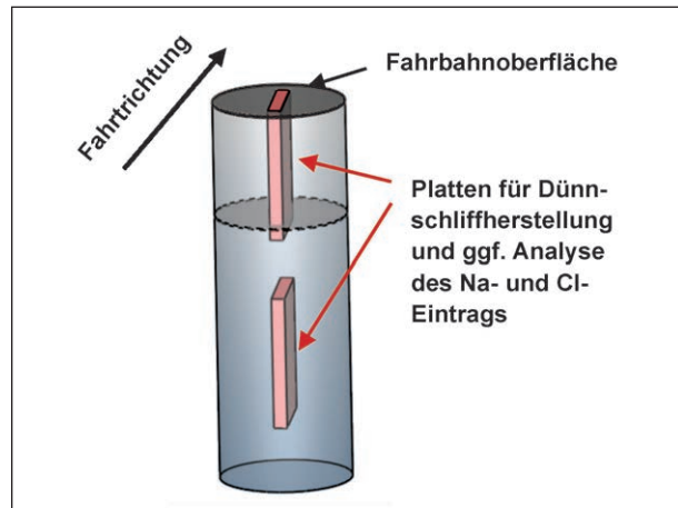
Bild 17: Räumliche Einordnung herausgearbeiteter Segmente aus dem Diagnosebohrkern aus dem Fugenkreuz der Fahrbahnplatte für die DS-Herstellung (Mikroskopie) und Analyse des Tausalzeintrags bei ein- und zweischichtiger Bauweise (Querscheinfuge links)
