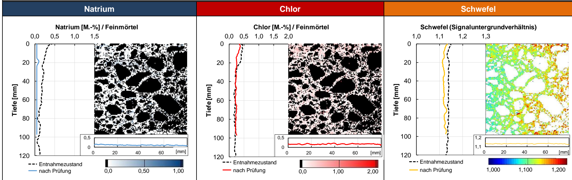
Abbildung 6.2c: Ergebnis der LIBS-Analyse – Probe aus Entnahmebereich BAB A14-GB-B (OB) nach 40 °C-Betonversuch –
