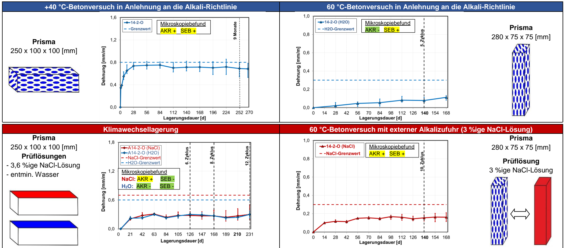
Abbildung 4.1: Ergebnisvergleich der Dehnungsmessungen aller AKR-provozierender Lagerungen mit Mikroskopiebefunden – Entnahmebereich A14-R2 (SK: III; Oberbeton) -
