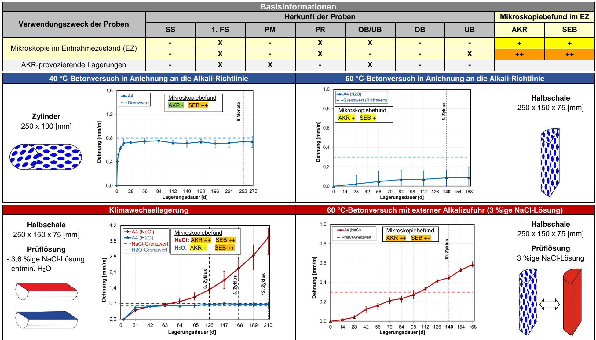
Abbildung 2.1: Ergebnisvergleich der Dehnungsmessungen aller AKR-provozierender Lagerungen mit Mikroskopiebefunden – Entnahmebereich A4 (SK: III) –
