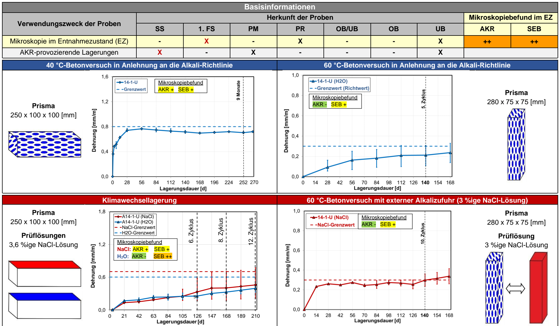
Abbildung 3.2: Ergebnisvergleich der Dehnungsmessungen aller AKR-provozierender Lagerungen mit Mikroskopiebefunden – Entnahmebereich A14-R1 (SK: II-III; Unterbeton) -
