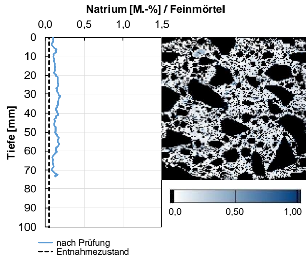
Abbildung 6.3d: Ergebnis der LIBS-Analyse – Probe aus Entnahmebereich BAB A14-GB-B (UB) nach 60 °C-Betonversuch –
