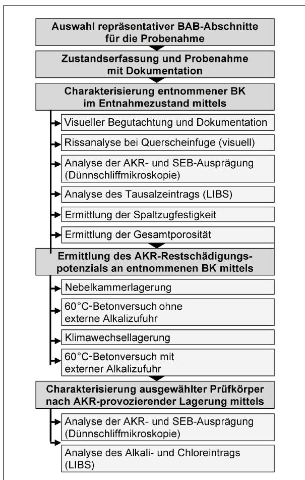
Bild 14: Vorgehensweise bei der Bewertung der AKR-Prüfverfahren (AP2)
