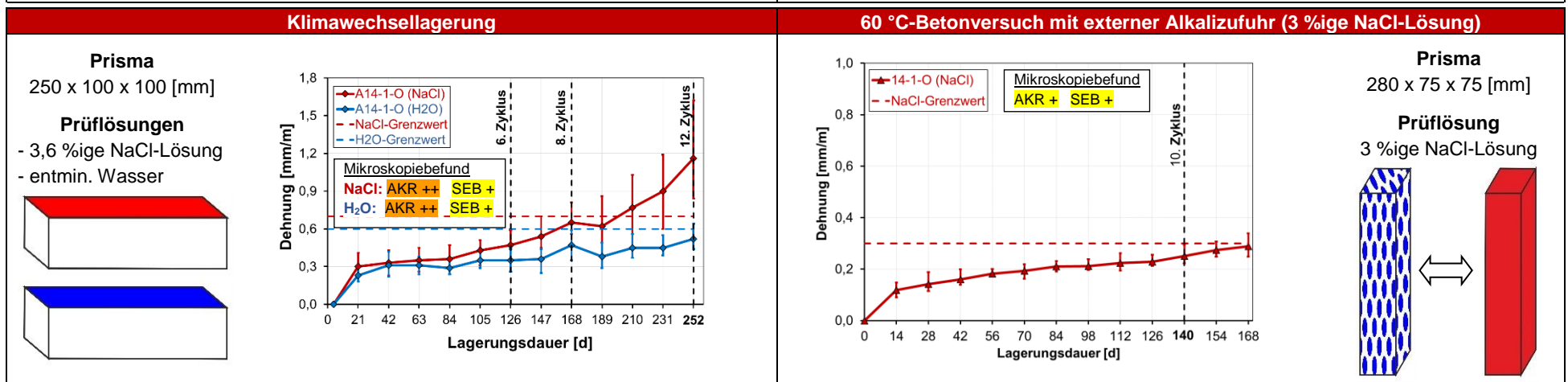
Abbildung 3.1: Ergebnisvergleich der Dehnungsmessungen aller AKR-provozierender Lagerungen mit Mikroskopiebefunden – Entnahmebereich A14-R1 (SK: II-III; Oberbeton) -
