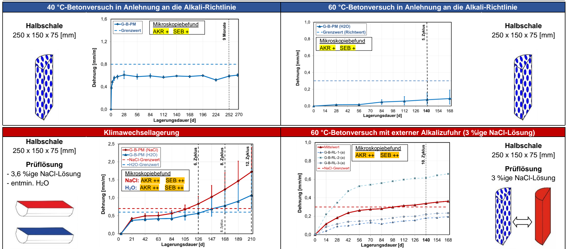
Abbildung 7.1: Ergebnisvergleich der Dehnungsmessungen aller AKR-provozierender Lagerungen mit Mikroskopiebefunden – Entnahmbereich A14-GB-B-PM (Entnahmejahr: 2014; SK: I-II; Ober- und Unterbeton) -
