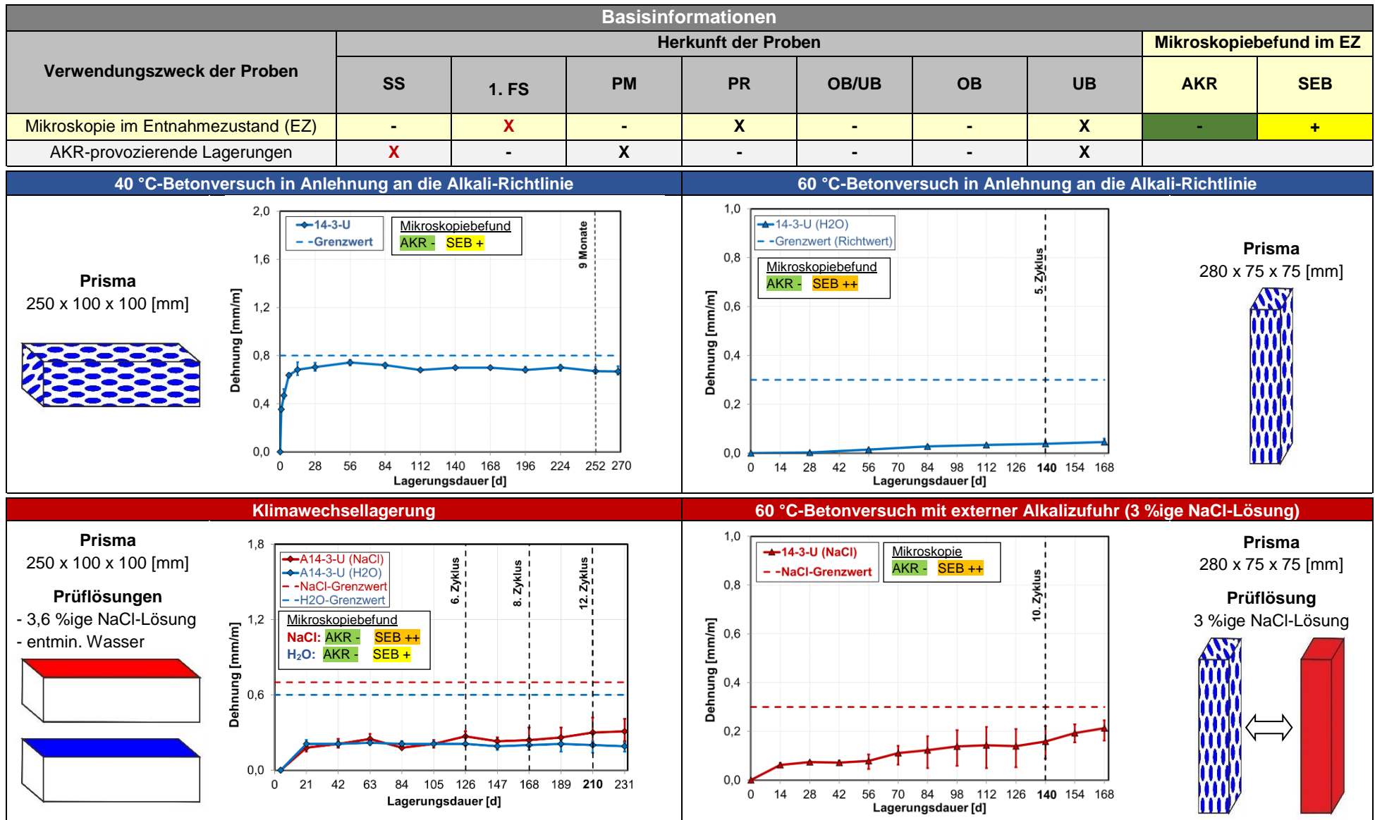
Abbildung 5.1: Ergebnisvergleich der Dehnungsmessungen aller AKR-provozierender Lagerungen mit Mikroskopiebefunden – Entnahmebereich A14-R3 (SK: III; Unterbeton) -
