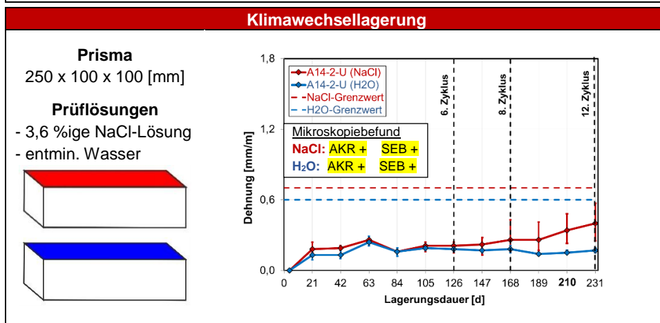
Abbildung 4.2: Ergebnisvergleich der Dehnungsmessungen aller AKR-provozierender Lagerungen mit Mikroskopiebefunden – Entnahmebereich A14-R2 (SK: III; Unterbeton) -
