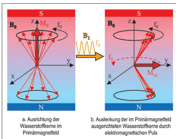
Bild 8: Schematische Darstellung des NMR-Messprinzips
