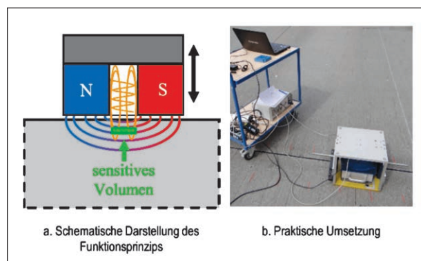
Bild 9: NMR-MOUSE
