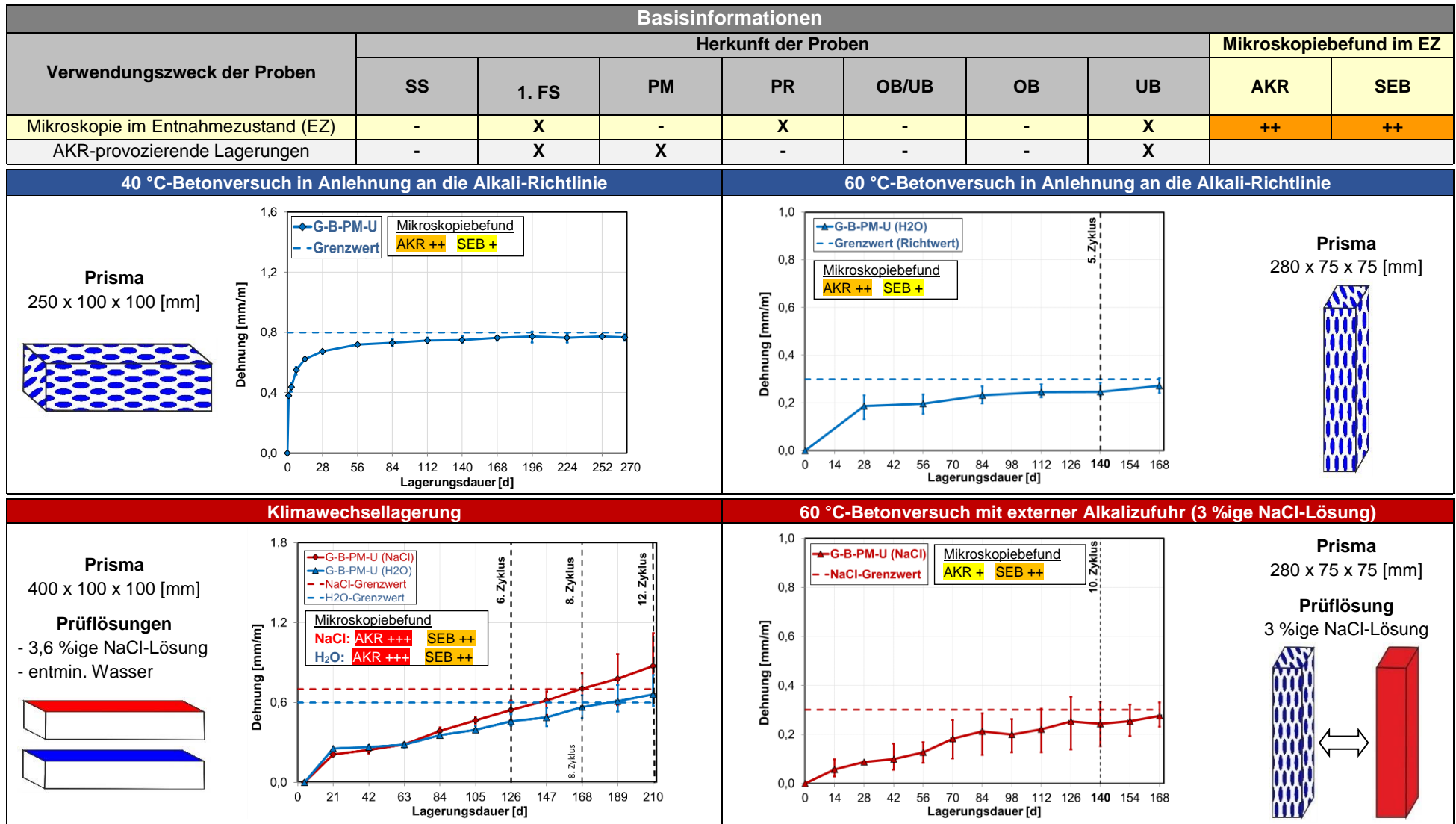
Abbildung 7.3: Ergebnisvergleich der Dehnungsmessungen aller AKR-provozierender Lagerungen mit Mikroskopiebefunden – Entnahmebereich A14-GB-B-PM (Entnahmejahr: 2014; SK: I-II; Unterbeton) -
