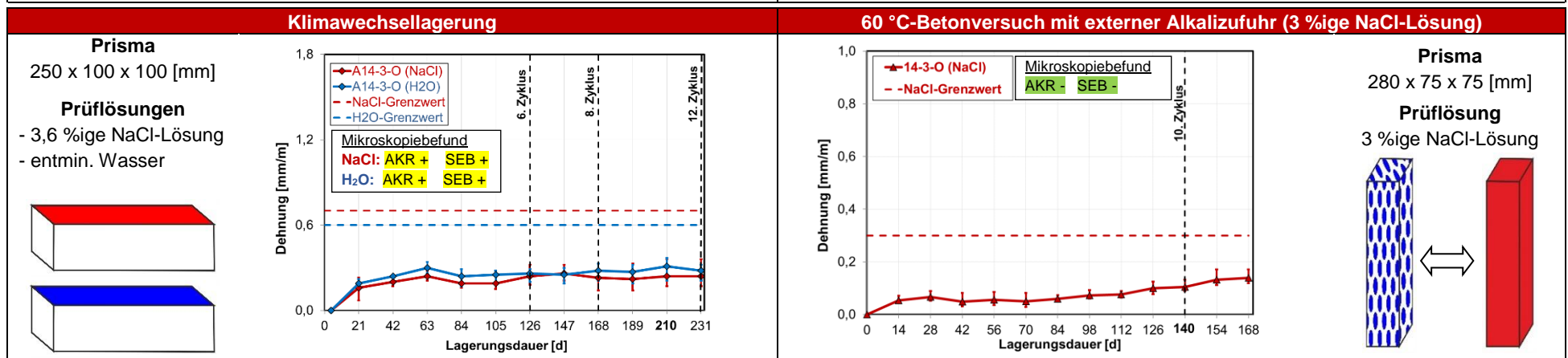
Abbildung 5.1: Ergebnisvergleich der Dehnungsmessungen aller AKR-provozierender Lagerungen mit Mikroskopiebefunden – Entnahmebereich A14-R3 (SK: III; Oberbeton) -
