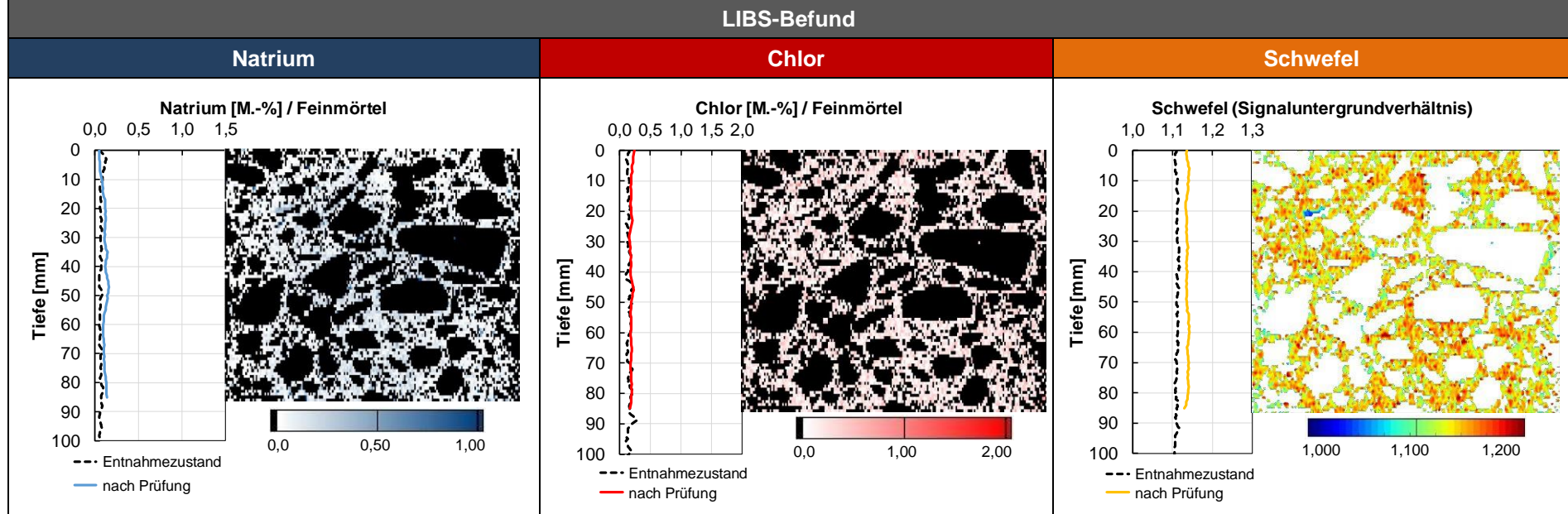
Abbildung 4.8: Ergebnis der LIBS-Analyse – Probe aus Entnahmebereich BAB A14-R3 (UB) nach 40 °C-Betonversuch –
