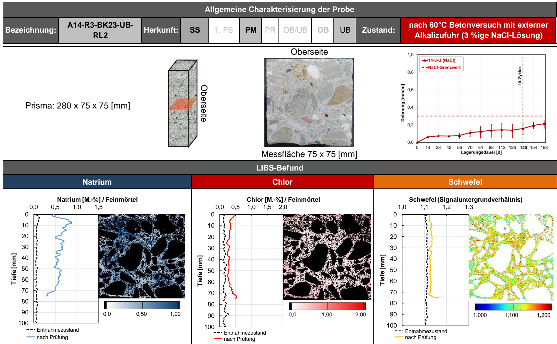
Abbildung 4.10: Ergebnis der LIBS-Analyse – Probe aus Entnahmebereich BAB A14-R3 (UB) nach 60 °C-Betonversuch mit externer Alkalizufuhr (3 %ige NaCl-Lösung) –
