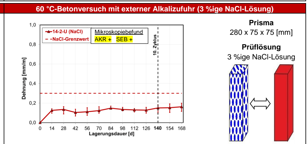
Abbildung 4.2: Ergebnisvergleich der Dehnungsmessungen aller AKR-provozierender Lagerungen mit Mikroskopiebefunden – Entnahmebereich A14-R2 (SK: III; Unterbeton) -
