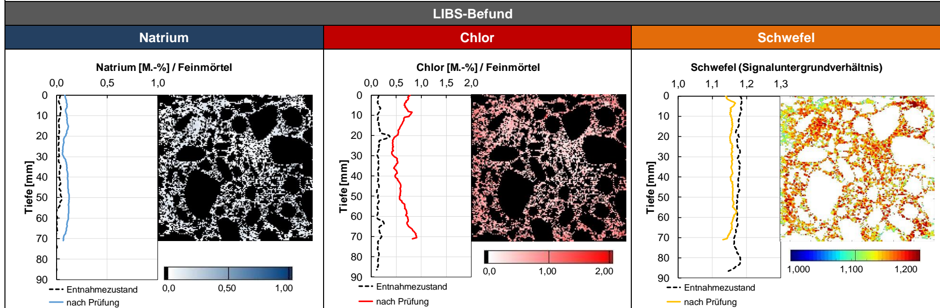
Abbildung 2.10: Ergebnis der LIBS-Analyse – Probe aus Entnahmebereich BAB A14-R1 (UB) nach 60 °C-Betonversuch mit externer Alkalizufuhr (3 %ige NaCl-Lösung) –
