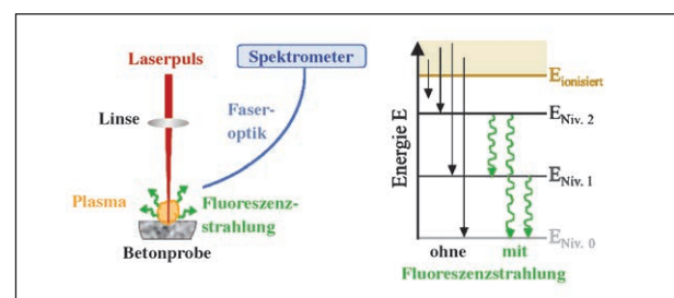
Bild 18: Schematische Darstellung des Messprinzips von LIBS
