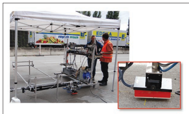
Bild 7: Vor Ort eingesetzter Bauwerksscanner für eine schnelle und automatisierte Durchführung der Radarmessung mit einem engen Messraster
