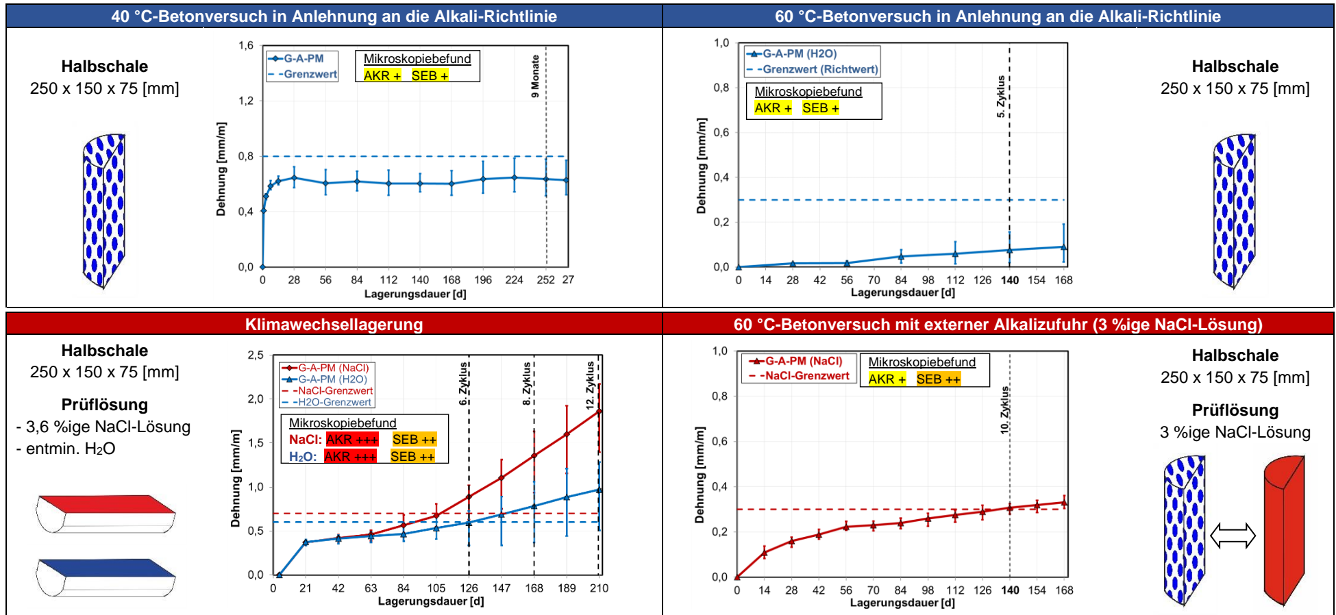
Abbildung 6.1: Ergebnisvergleich der Dehnungsmessungen aller AKR-provozierender Lagerungen mit Mikroskopiebefunden – Entnahmebereich A14-GB-A-PM (Entnahmejahr: 2010; SK: 0-I; Ober- und Unterbeton) -
