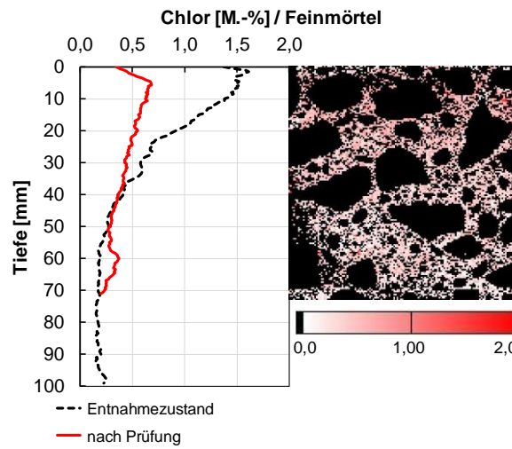
Abbildung 2.3: Ergebnis der LIBS-Analyse – Probe aus Entnahmebereich BAB A14-R1 nach 60 °C-Betonversuch –
