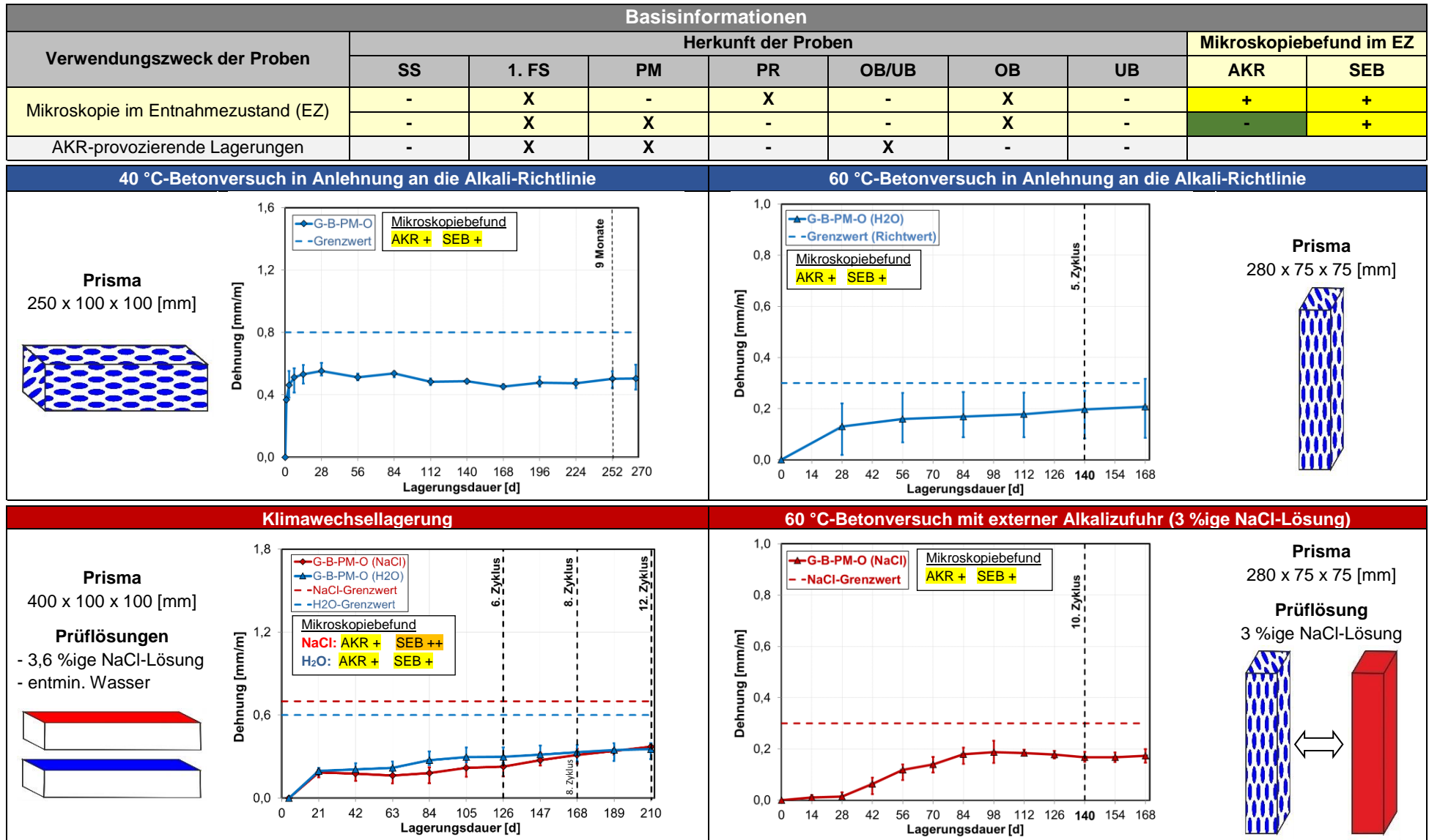
Abbildung 7.2: Ergebnisvergleich der Dehnungsmessungen aller AKR-provozierender Lagerungen mit Mikroskopiebefunden – Entnahmebereich A14-GB-B-PM (Entnahmejahr: 2014; SK: I-II; Oberbeton) -
