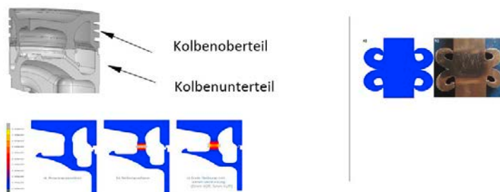
Abb. 8: Reibschweißvorgang, oben links: Übersicht, oben rechts: Evaluierung der vorhergesagten Reibschweißnaht (Wulstausbildung), unten: ausgewählte Phasen des Reibschweißprozesses
