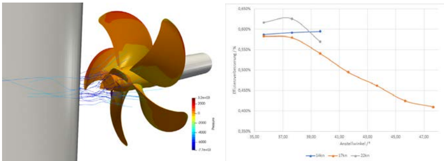
Abb. 6: Visualisierung der nabennahen Strömung für die optimierte Nabenkappenflosse (links) und Darstellung der Effizienzverbesserung bei einer Parametervariation für signifikante Geschwindigkeiten des Betriebsprofils (rechts).
