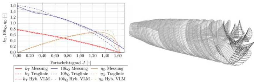
Abb. 5: Berechnete Freifahrt im Vergleich zur Messung für den EPROSYS Tandem-Propeller (links) und freies Wirbelsystem beider Propeller für J=1,0 (rechts).
