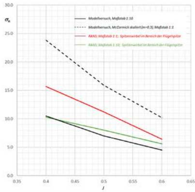
Abb. 6: Kavitationszahl \sigma_n in Abhängigkeit der Fortschrittsziffer und des Maßstabes
