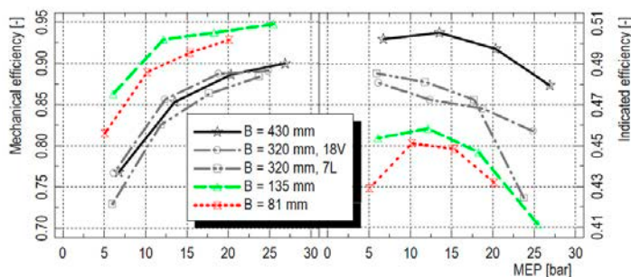
Abb. 1: Vergleich von mechanischen und indizierten Wirkungsgraden verschiedener Motorengrößen [2]
