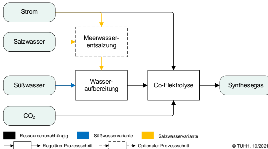
Abbildung 3-12 Schematische Darstellung der Synthesegaserzeugung mittels Co-Elektrolyse
