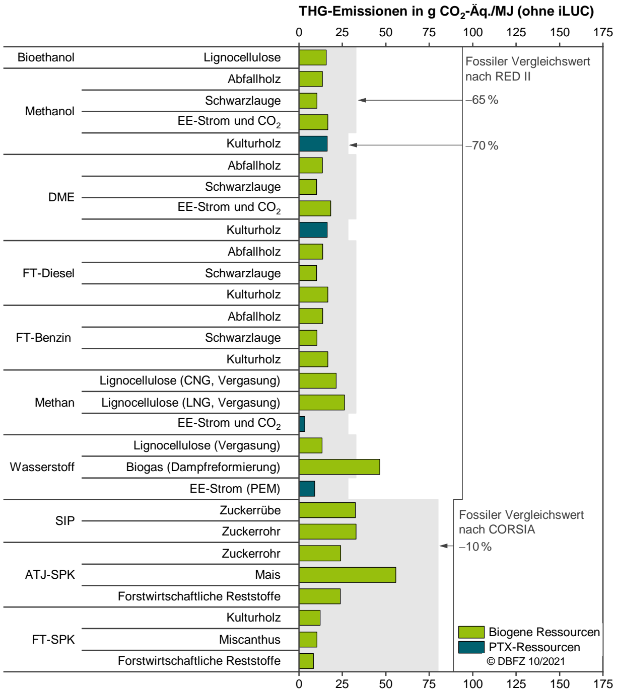
Abbildung 7-3 THG-Emissionen kommender Energieträger, Datenbasis: [Alamia (2017); 37. BImSchV (2017); Bongartz; Bongartz (2018); Richtlinie (EU) 2018/2001 (2018); Hajjaji (2016); ISCC System GmbH (2020b)]
