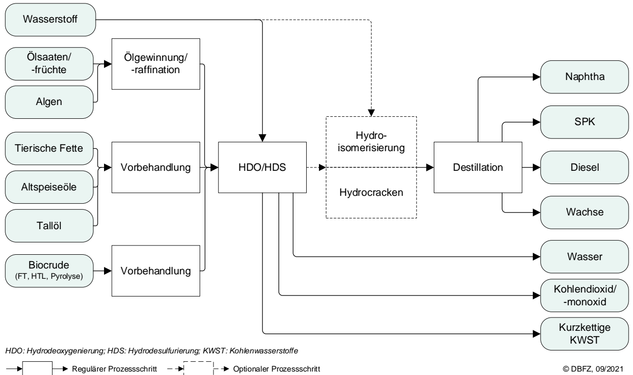
Abbildung 3-7 Schematische Darstellung der Produktion von HVO/HEFA-Kraftstoffen
