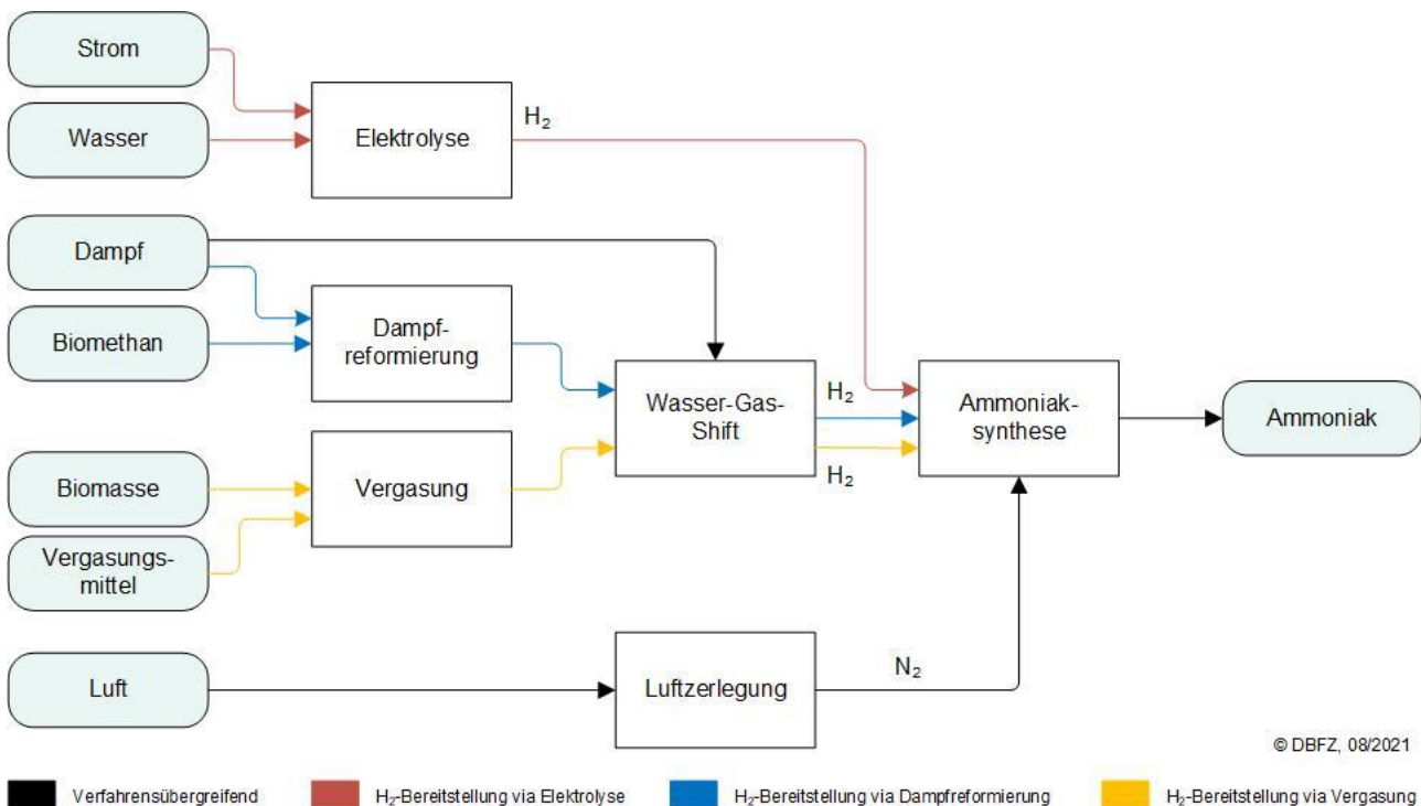
Abbildung 3-14 Verfahren zur Herstellung von Ammoniak unter Verwendung von biogenen Ressourcen
