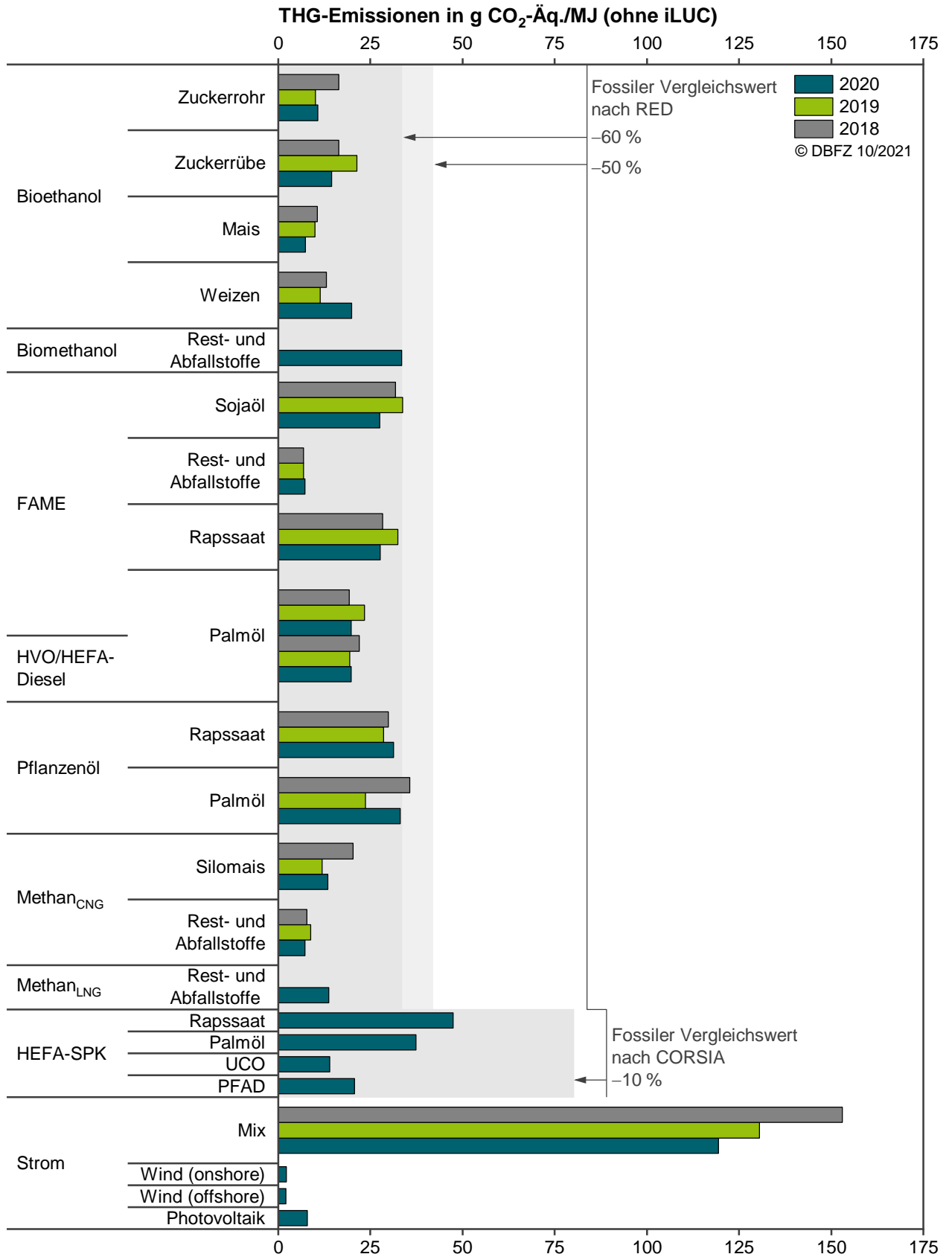
Abbildung 7-2 THG-Emissionen kommerziell verfügbarer Kraftstoffe, Hinweis: Methan aus Vergärung, Die angegebenen THG-Emissionen entsprechen den Werten, die beim Antrag zur Anrechnung auf die THG-Quote bei der BLE in einem Berichtsjahr angegeben wurden. Sie sind nicht als typische Werte für die jeweilige Biokraftstoffart zu
