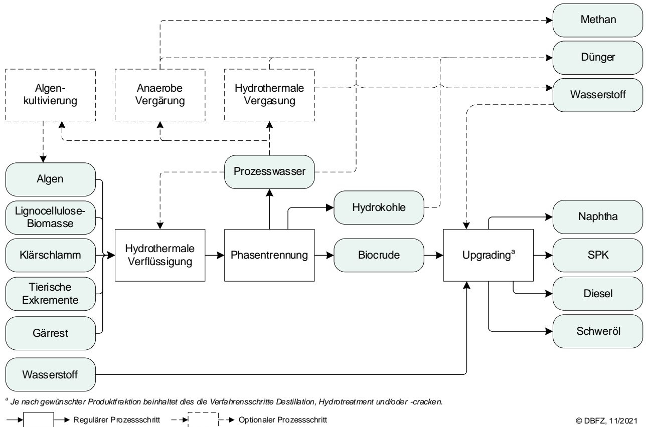
Abbildung 3-8 Schematische Darstellung der Produktion von HTL-Kraftstoffen
