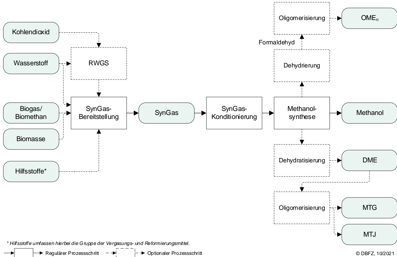
Abbildung 3-13 Schematische Darstellung der Methanolsynthese und ausgewählter Folgetechnologien
