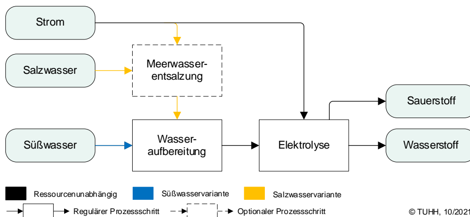
Abbildung 3-10 Schematische Darstellung der Elektrolyseverfahren aus Salz- bzw. Süßwasser zur Produktion von Wasserstoff
