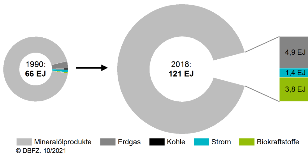
Abbildung 5-1 Weltweiter Endenergieverbrauch im Verkehrssektor nach Energiequellen in den Jahren 1990 und 2018, Datenbasis: [IEA (2021b), (2021d)]
