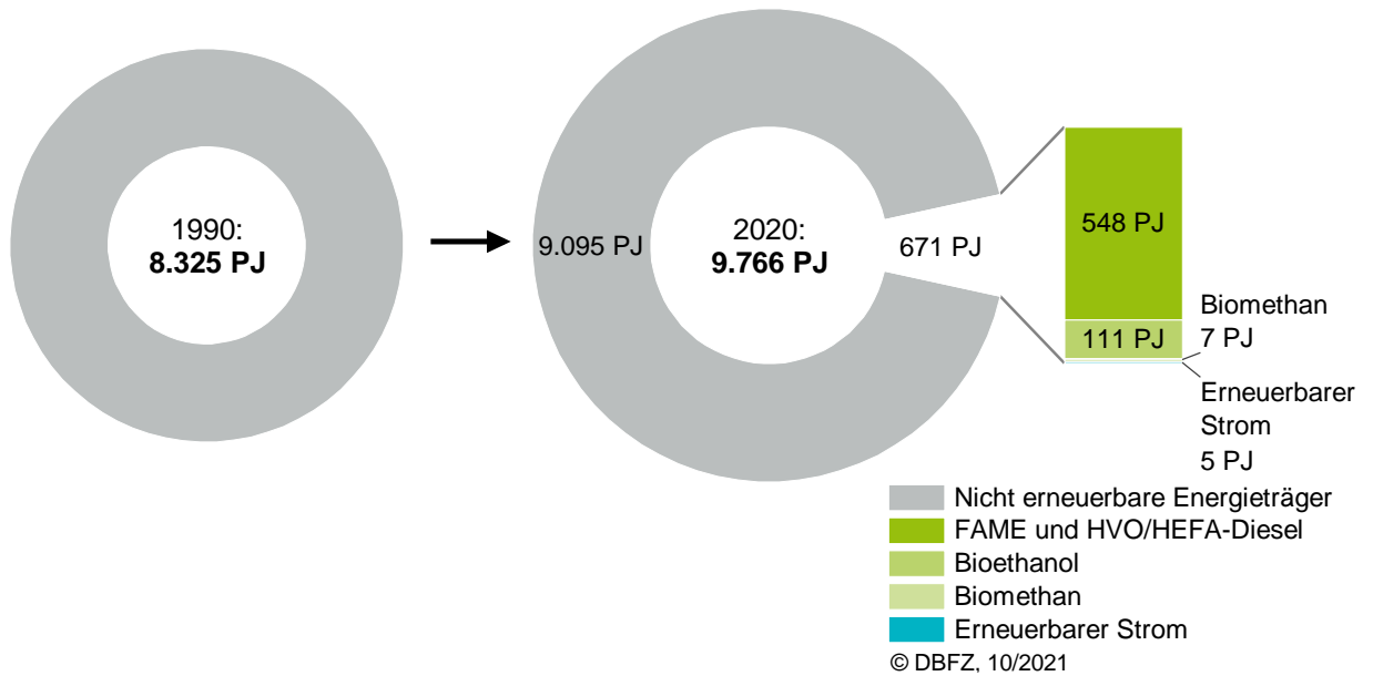
Abbildung 5-22 Nutzung von nicht erneuerbaren und erneuerbaren Energieträgern im Straßenverkehr der Europäischen Union, Hinweis: EU-27, Datenbasis: [Eurostat (2021c)]
