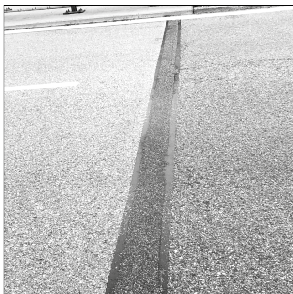
Bild 85: Schadensfreie Belagsdehnfuge der Brücke im Zuge der BAB A 95 nach 5 Jahren unter Verkehr (6)
