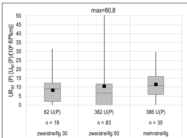
Bild 3-41: Bandbreite der Unfallrate von Radverkehrsunfällen auf Streckenabschnitten
