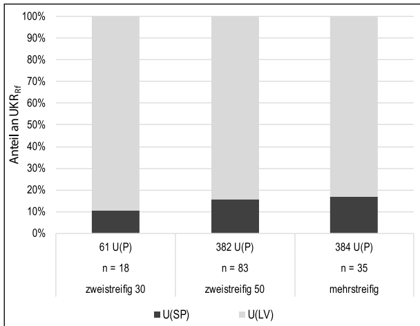
Bild 3-44: Anteile der Unfälle mit schwerem und leichtem Personenschaden an den mittleren Unfallkostenraten auf Streckenabschnitten je Streckentyp für Unfälle mit Personenschaden und Radverkehrsbeteiligung
