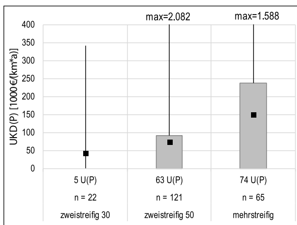
Bild 3-52: Bandbreite der Unfallkostendichte von Radverkehrsunfällen in Annäherungsbereichen von HVKP je Streckentyp
