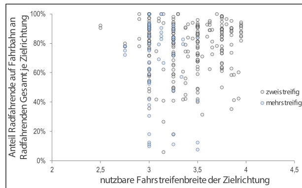
Bild 3-33: Anteil der Radfahrenden auf der Fahrbahn an allen Radfahrenden der Zielrichtung im Vergleich mit der nutzbaren Fahrstreifenbreite der Zielrichtung, n=296 Zielrichtungen
