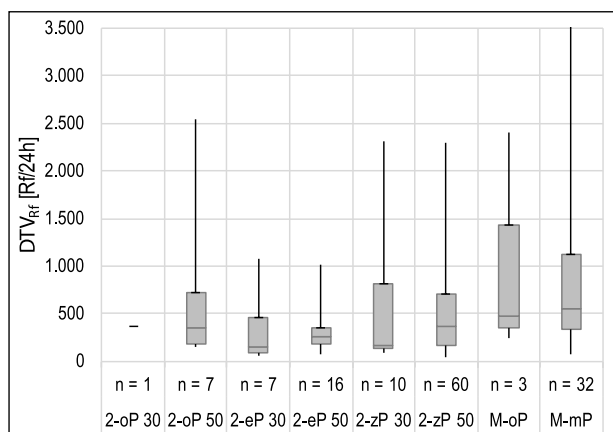
Bild 3-19: Bandbreiten der durchschnittlichen täglichen Verkehrsstärke des Radverkehrs nach Streckentyp. n entspricht der Anzahl der Untersuchungsstellen. Maximalwert für M-mP liegt bei 3628 Rf/24h (nicht angezeigt)
