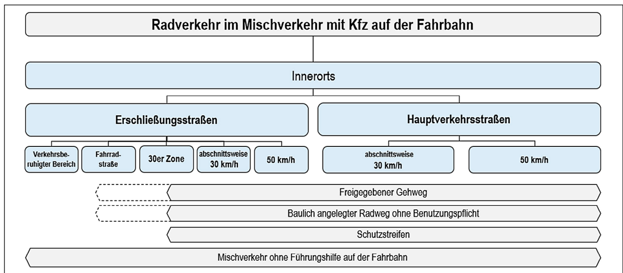
Bild 2-2: Verkehrstechnische Randbedingungen für verschiedene Umsetzungen des Radverkehrs im Mischverkehr mit Kfz auf der Fahrbahn auf Strecken zwischen Hauptverkehrsknotenpunkten (HVKP)
