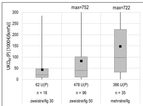
Bild 3-42: Bandbreite der Unfallkostendichte von Radverkehrsunfällen auf Streckenabschnitten je Streckentyp
